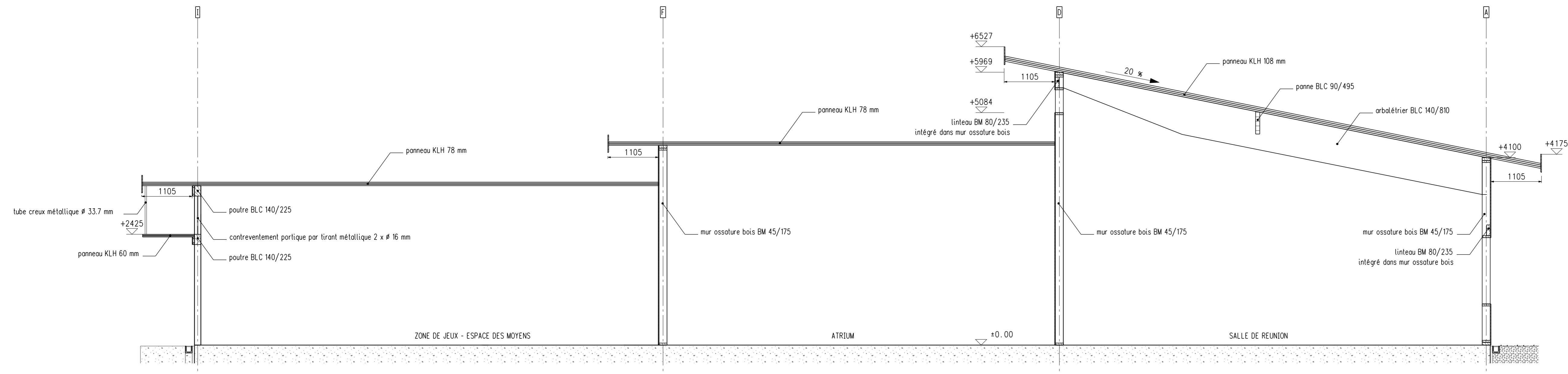
COUPE A-A
