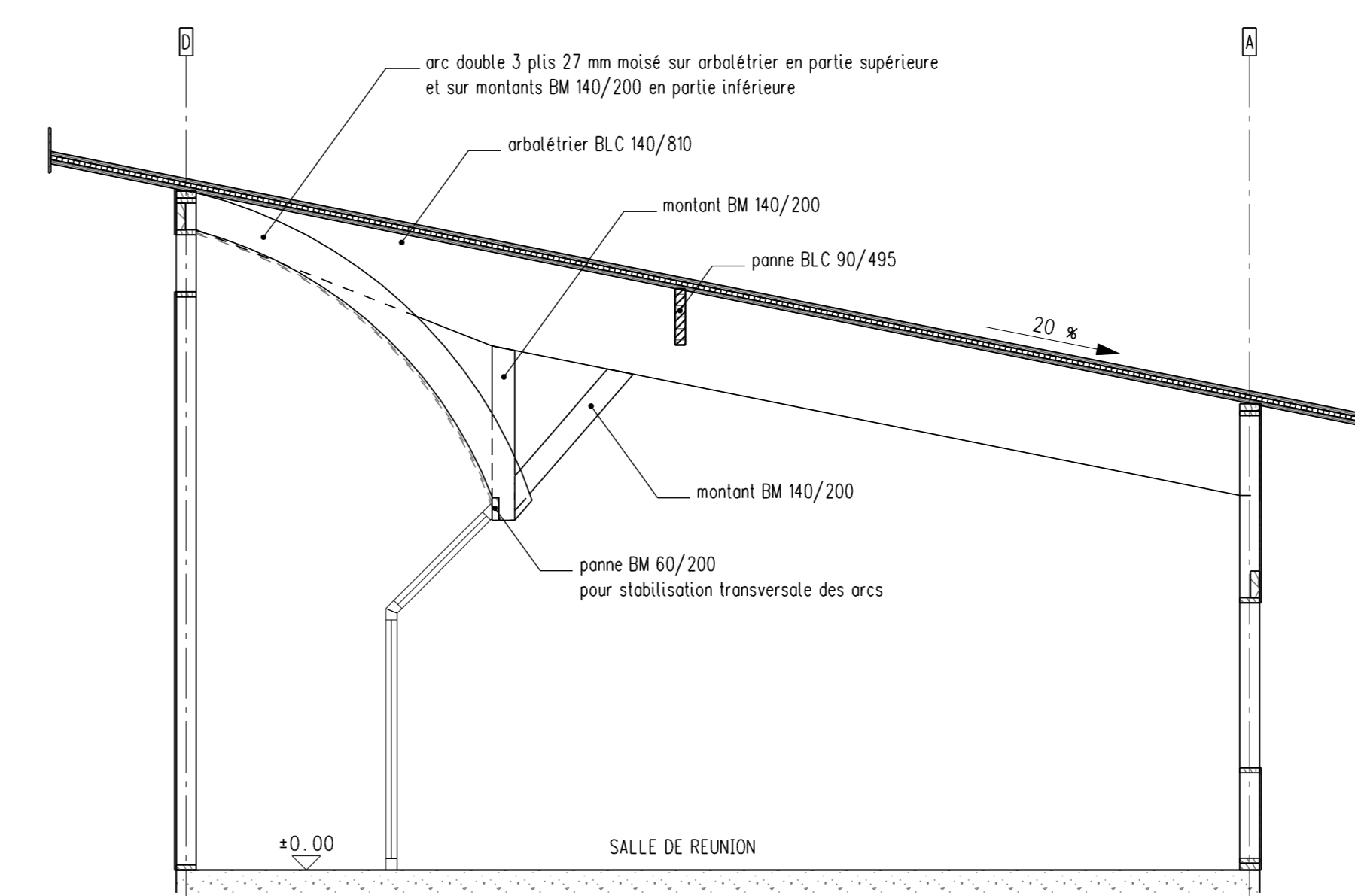
Coupe de principe support plafond cintré Cas de fixation sur arbalétrier
