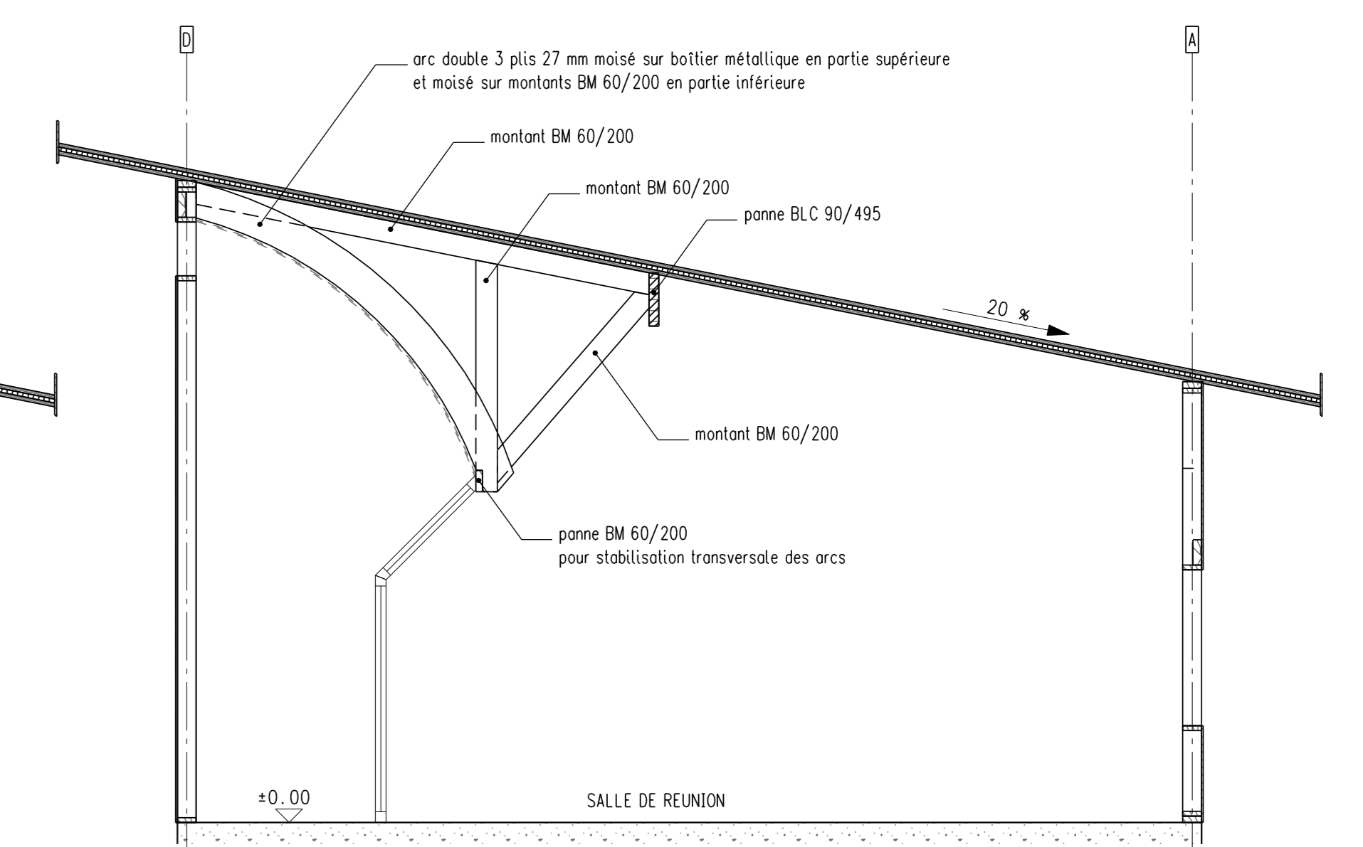
Coupe de principe support plafond cintré Cas courant
