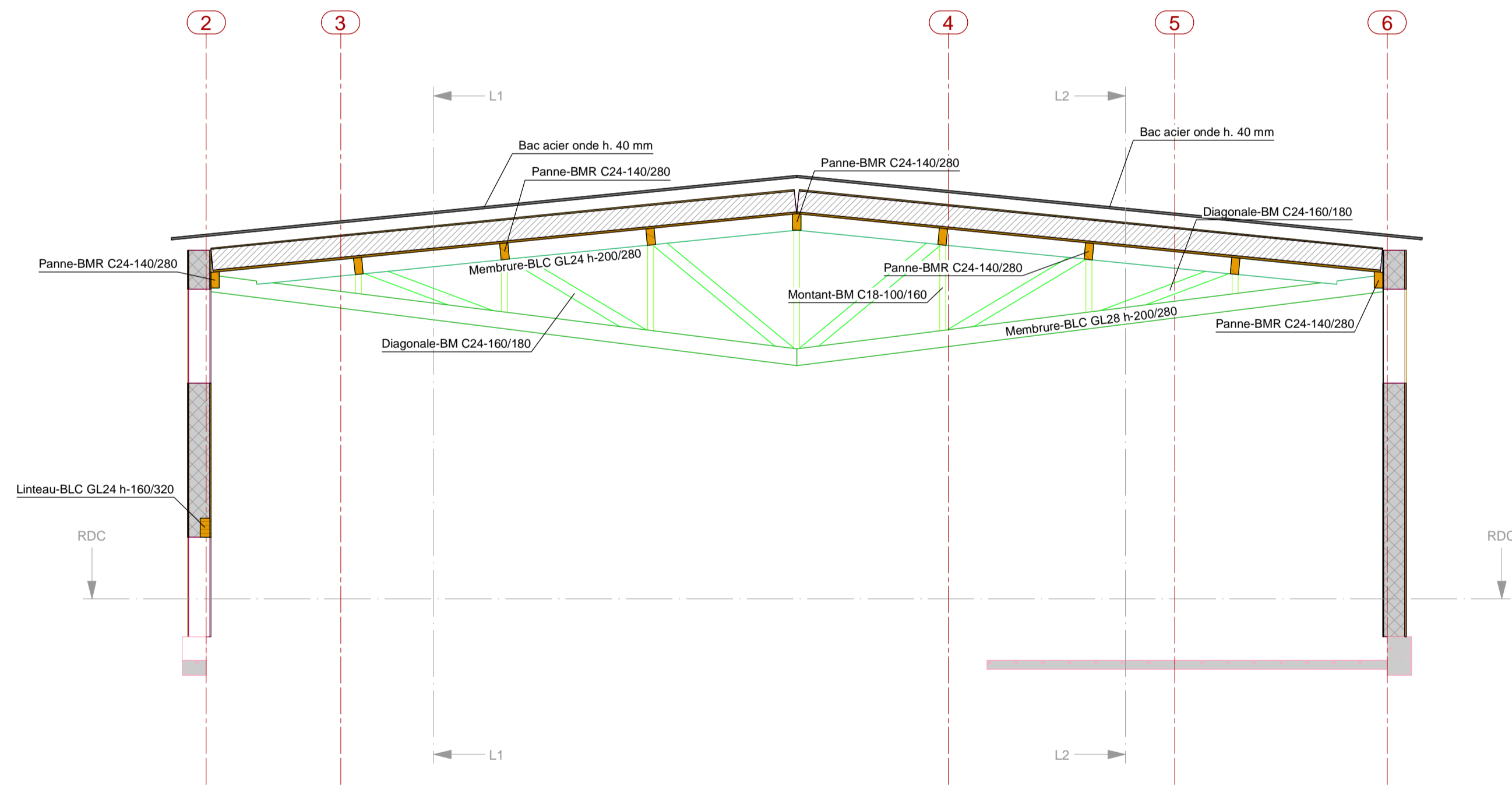
COUPE TRANSVERSALE T2
