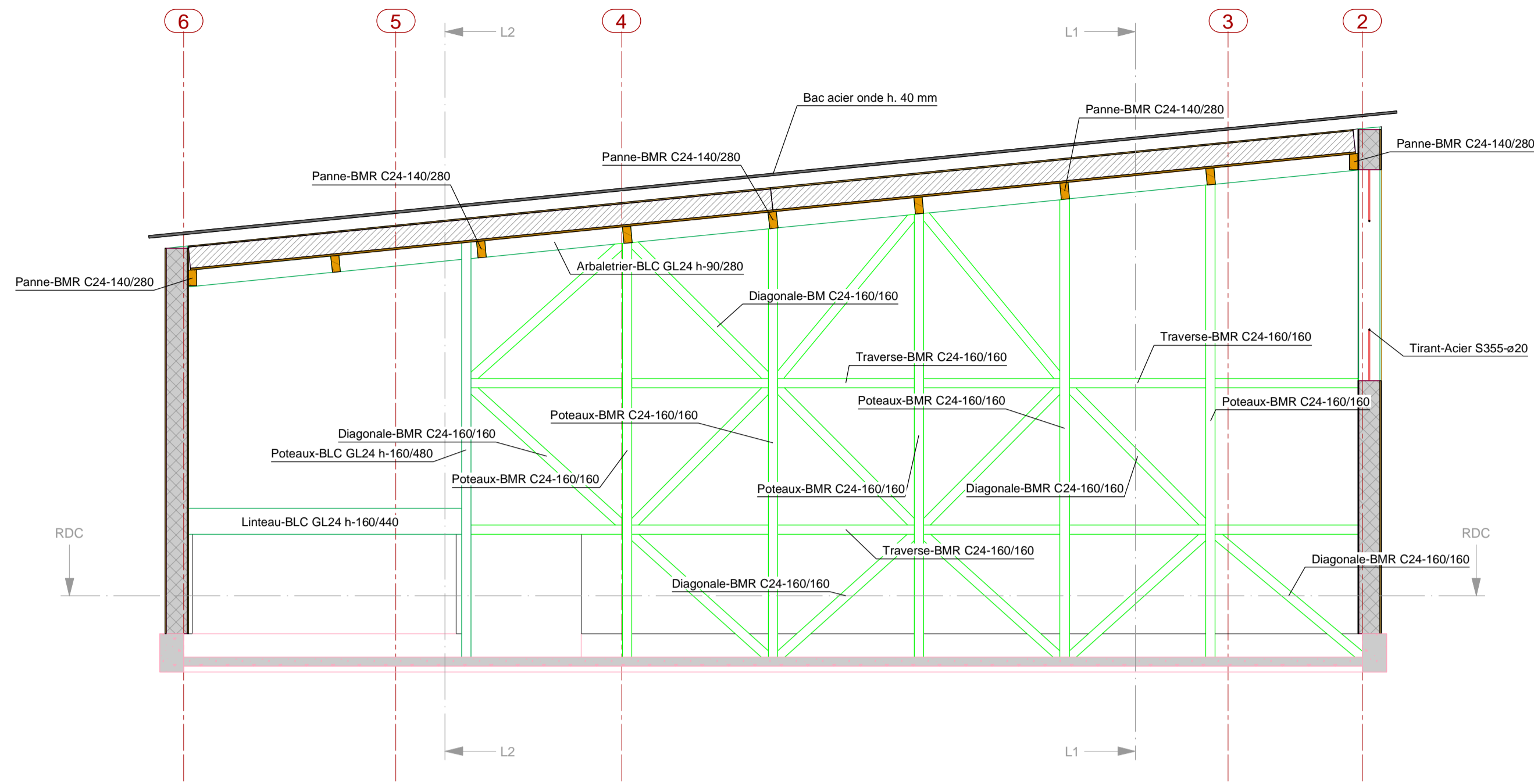
COUPE TRANSVERSALE T1
