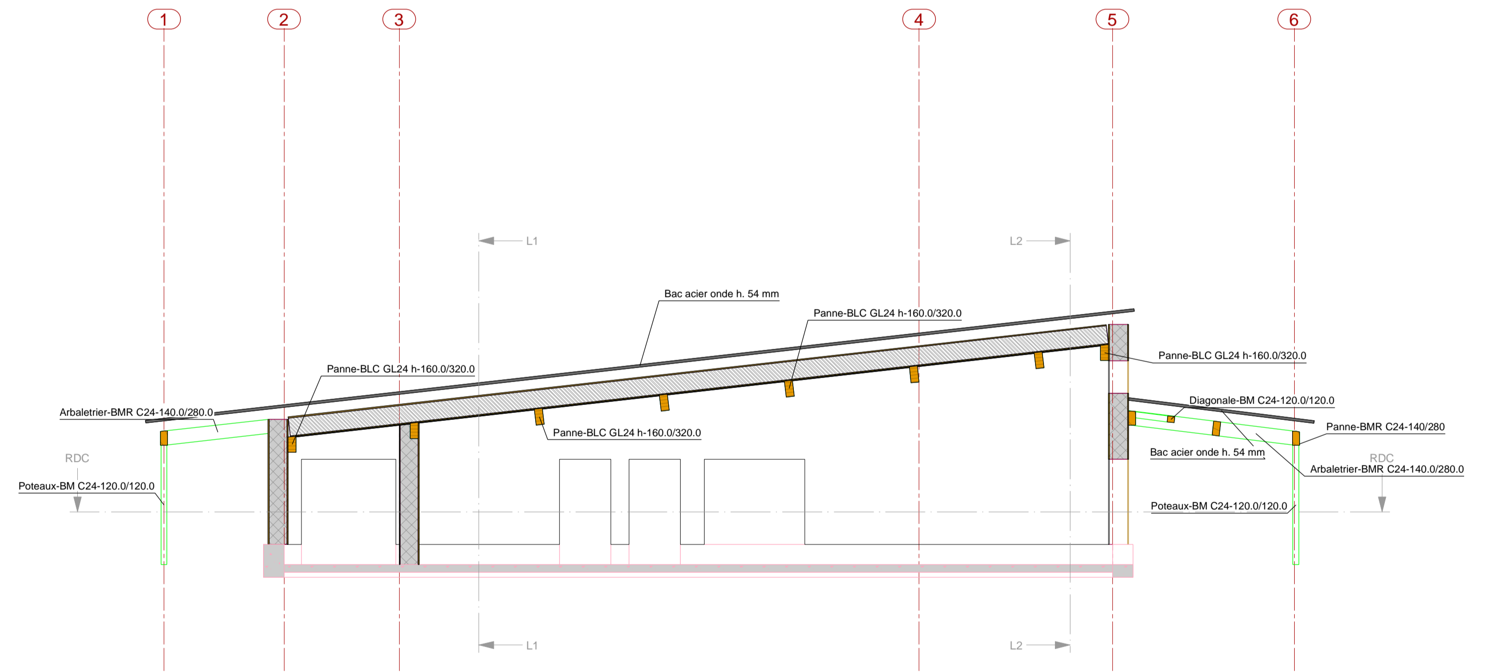
COUPE TRANSVERSALE T4
