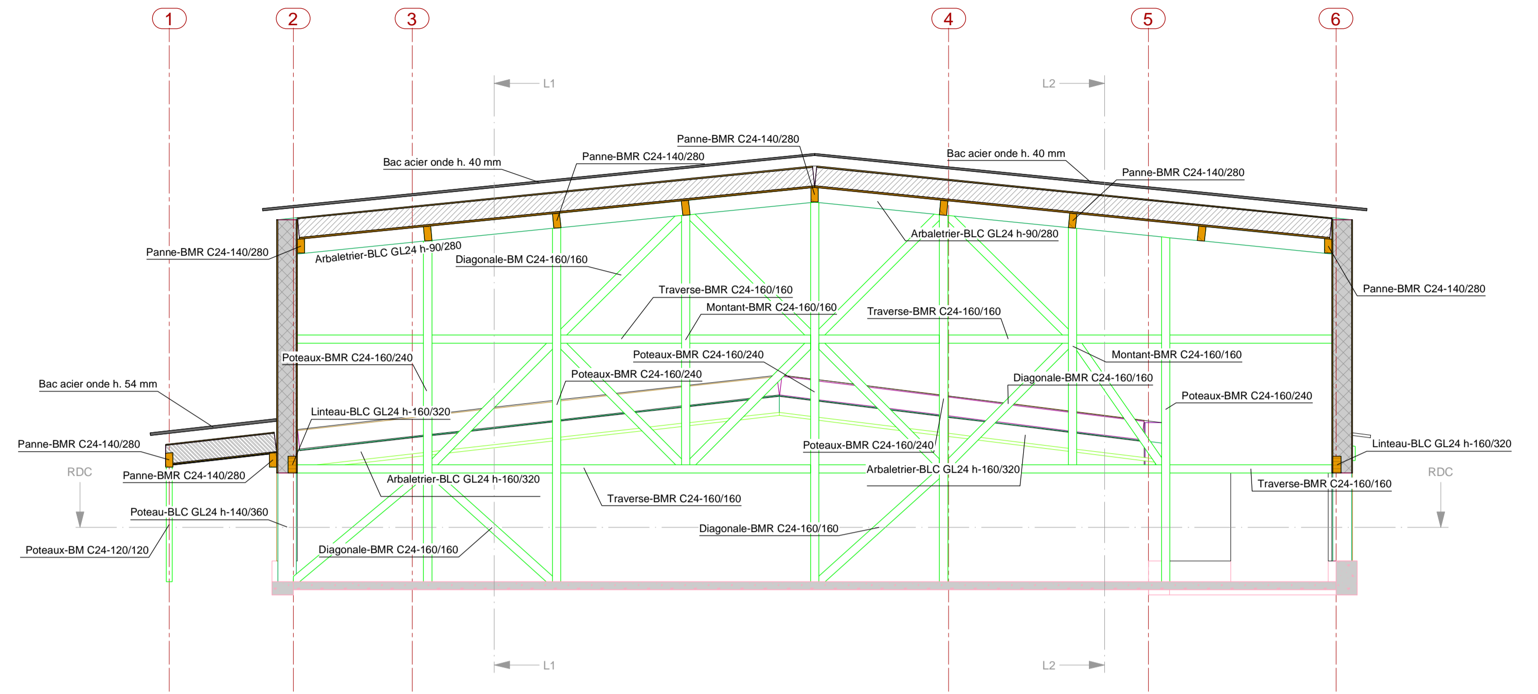
COUPE TRANSVERSALE T3
