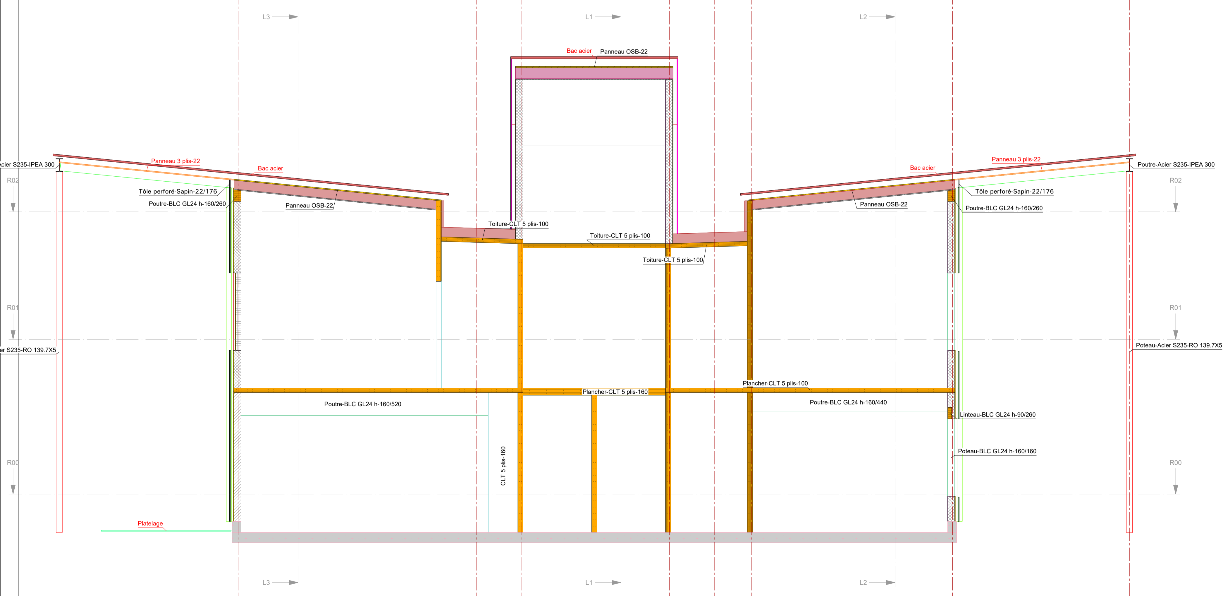
Coupe: T2-T2
