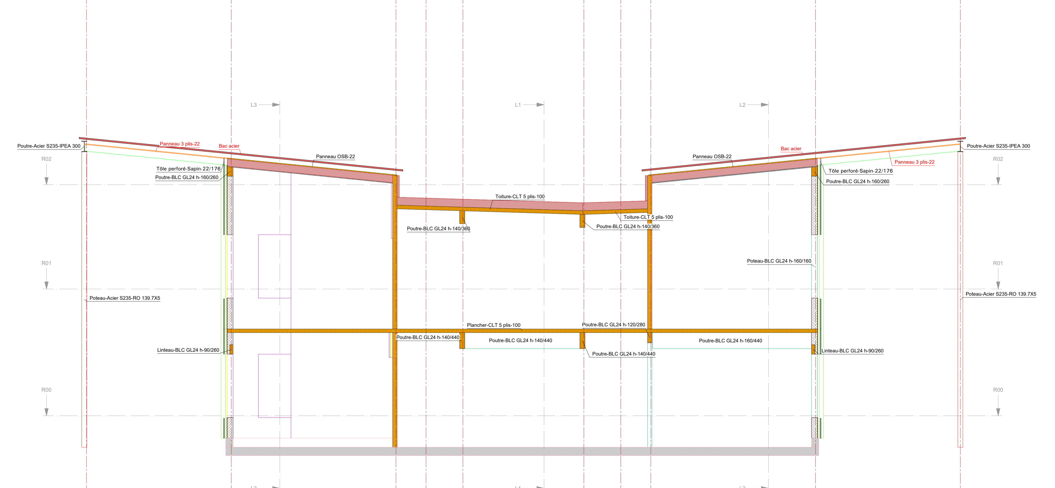
Coupe: T4-T4
