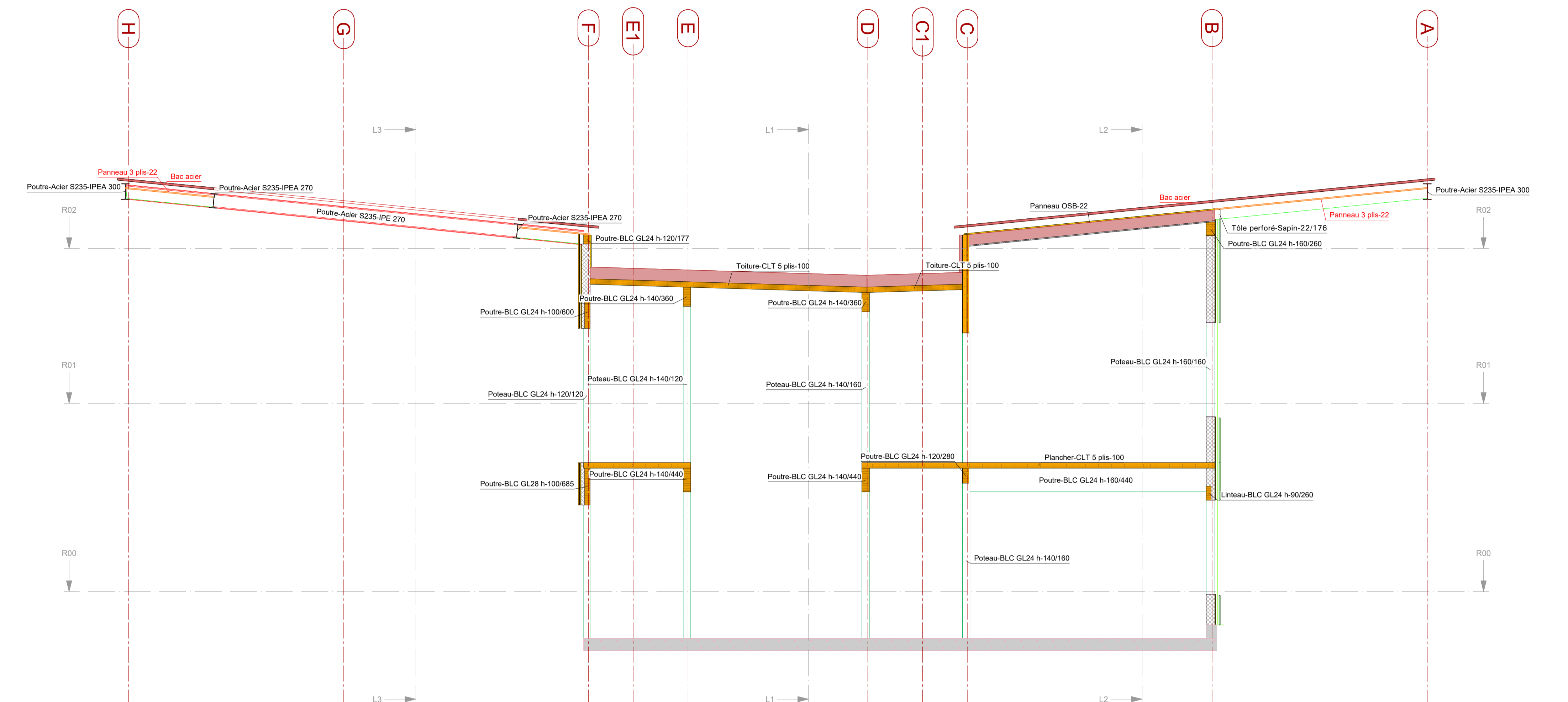
Coupe: T3-T3
