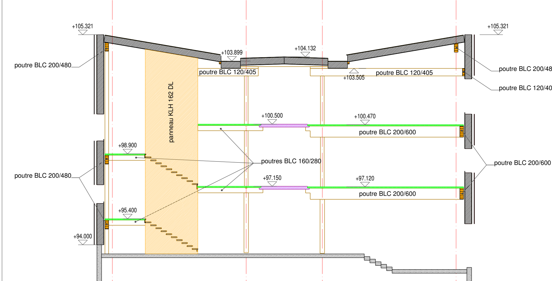
Coupe A
