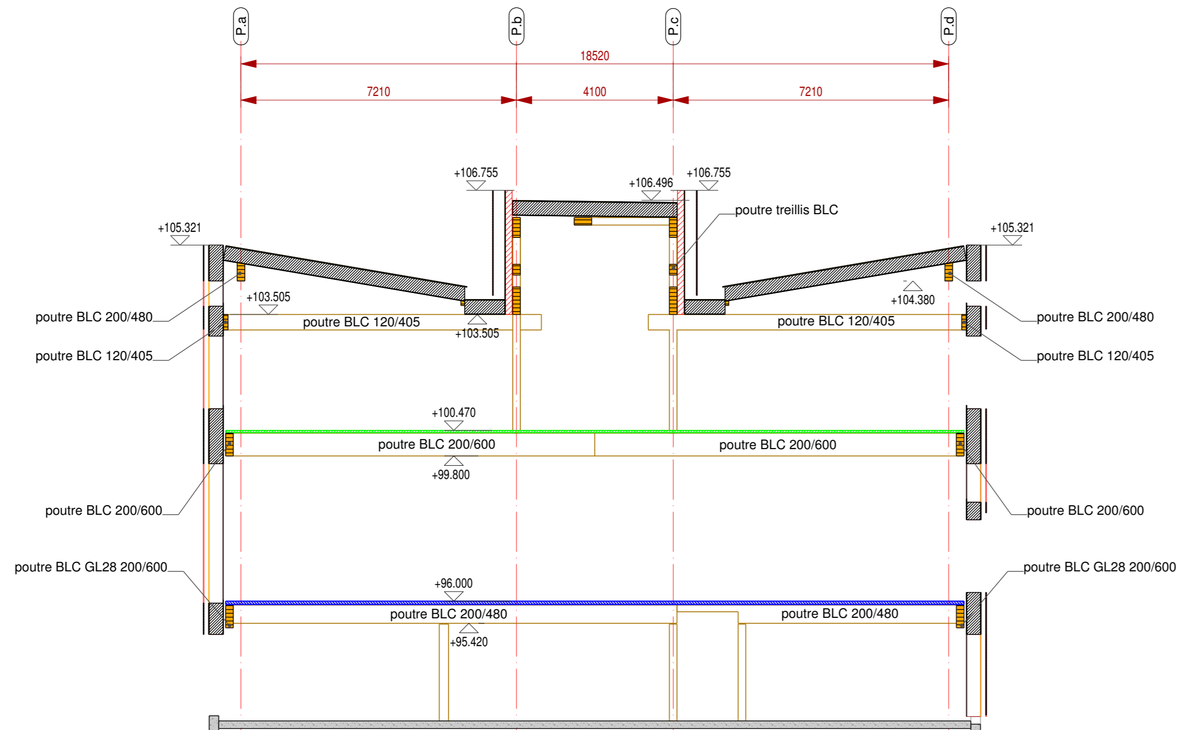
Coupe G
