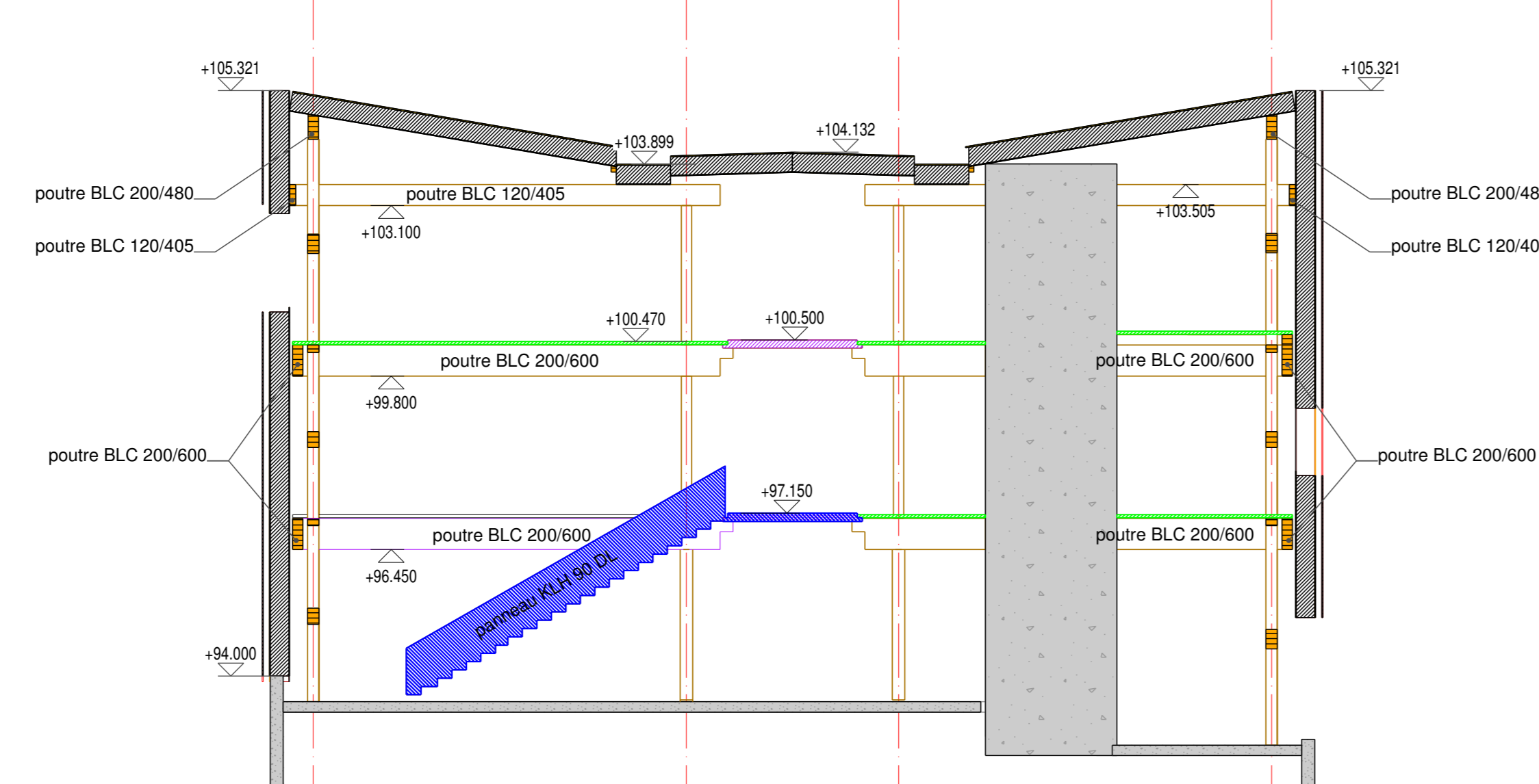
Coupe C
