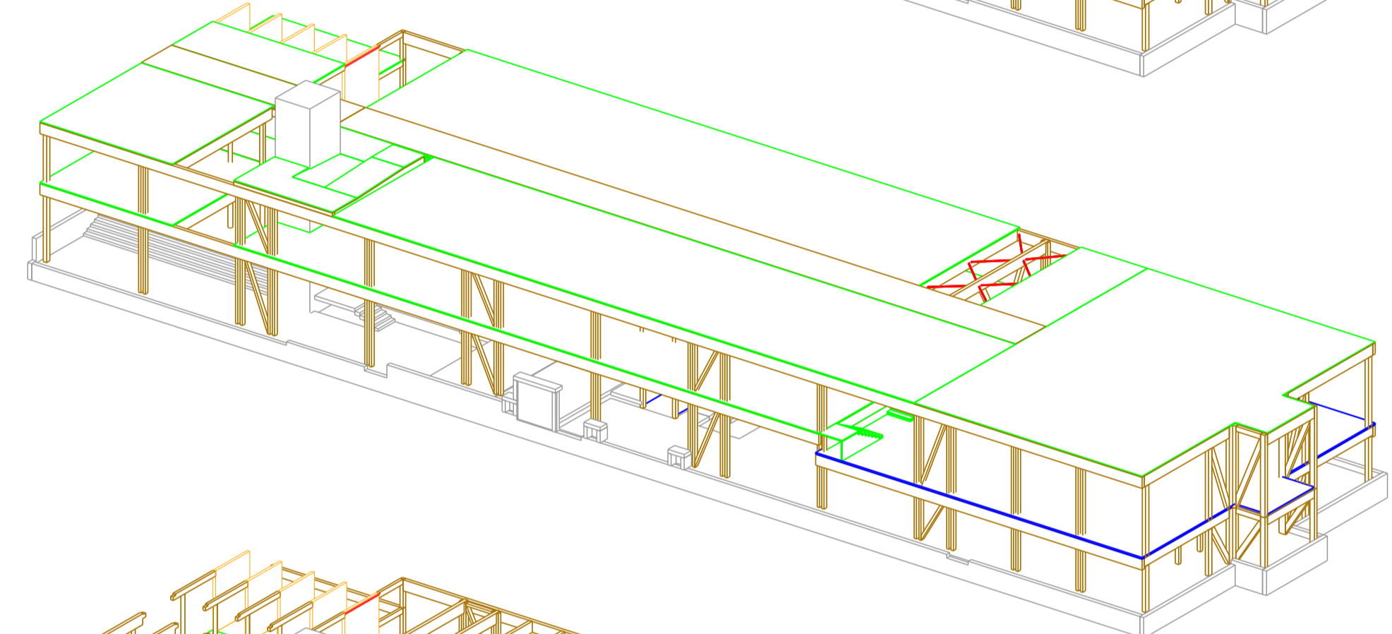
Plancher bas R+2
