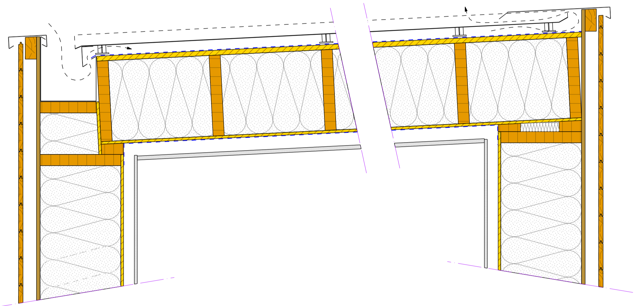
Coupe longitudinale de détail (1/10e)
