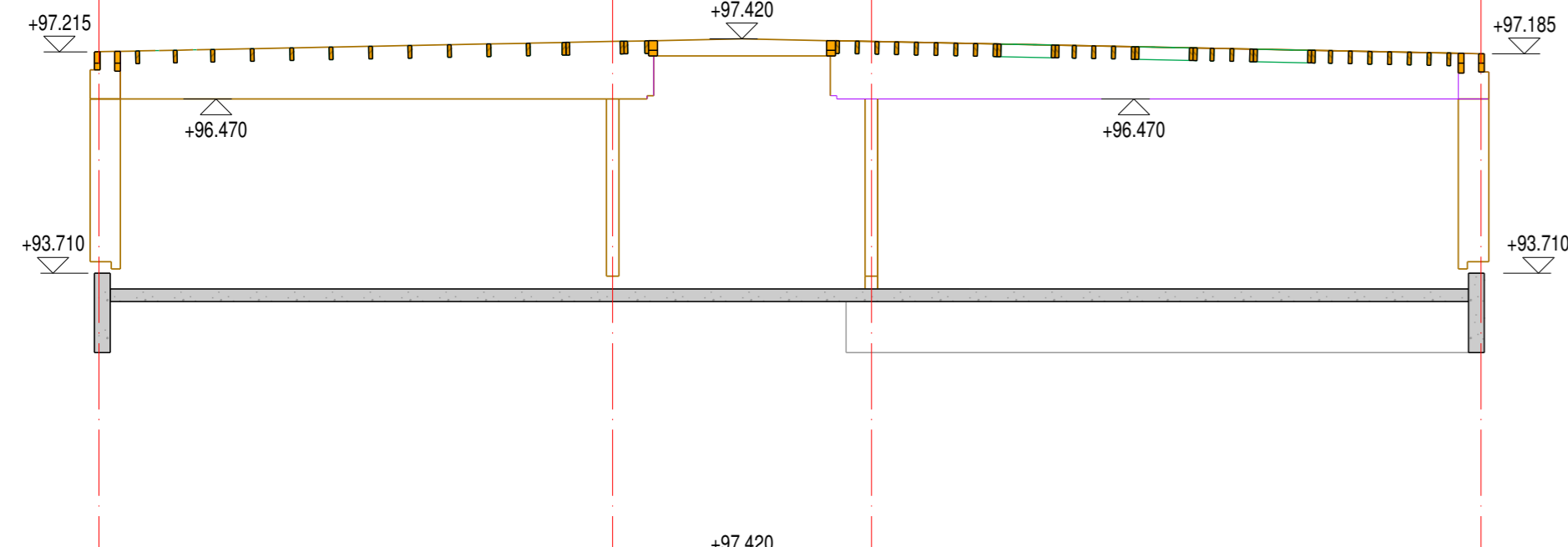
Coupe C
