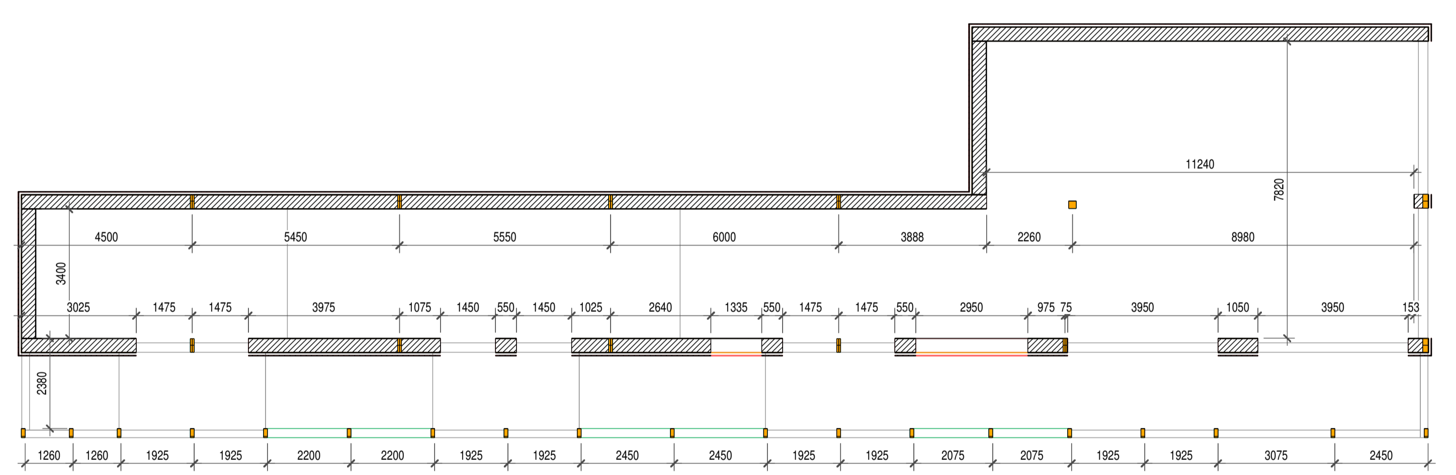
Plan d'implantation (1/100e)
