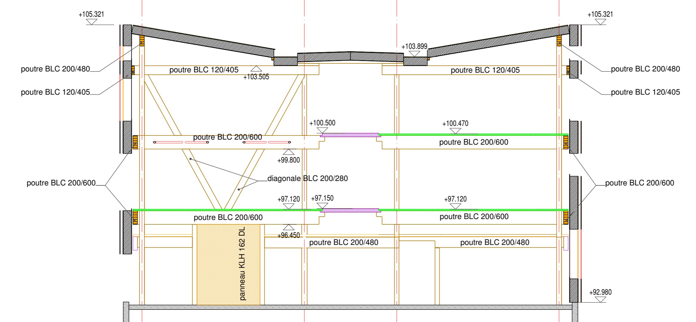
Coupe F
