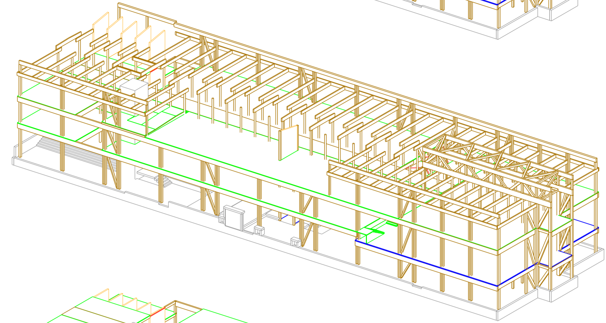
Structure bois R+2 et charpente
