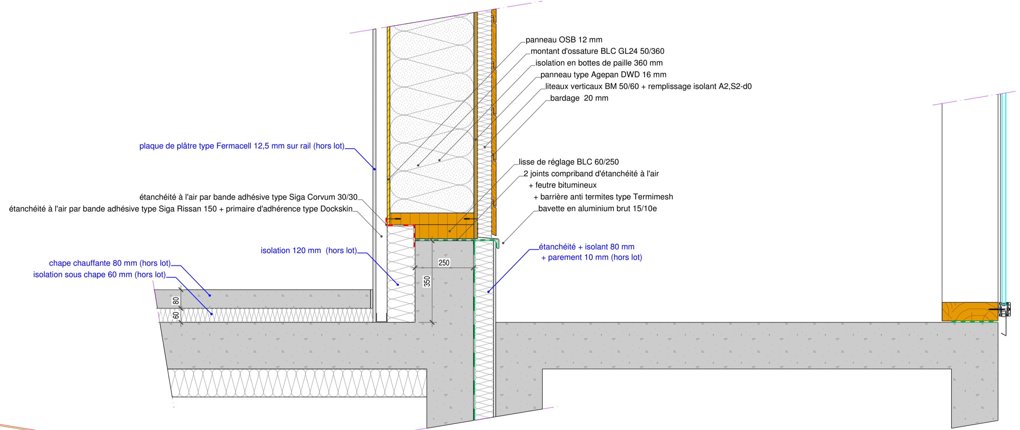
Coupe transversale de détail (1/10e)
