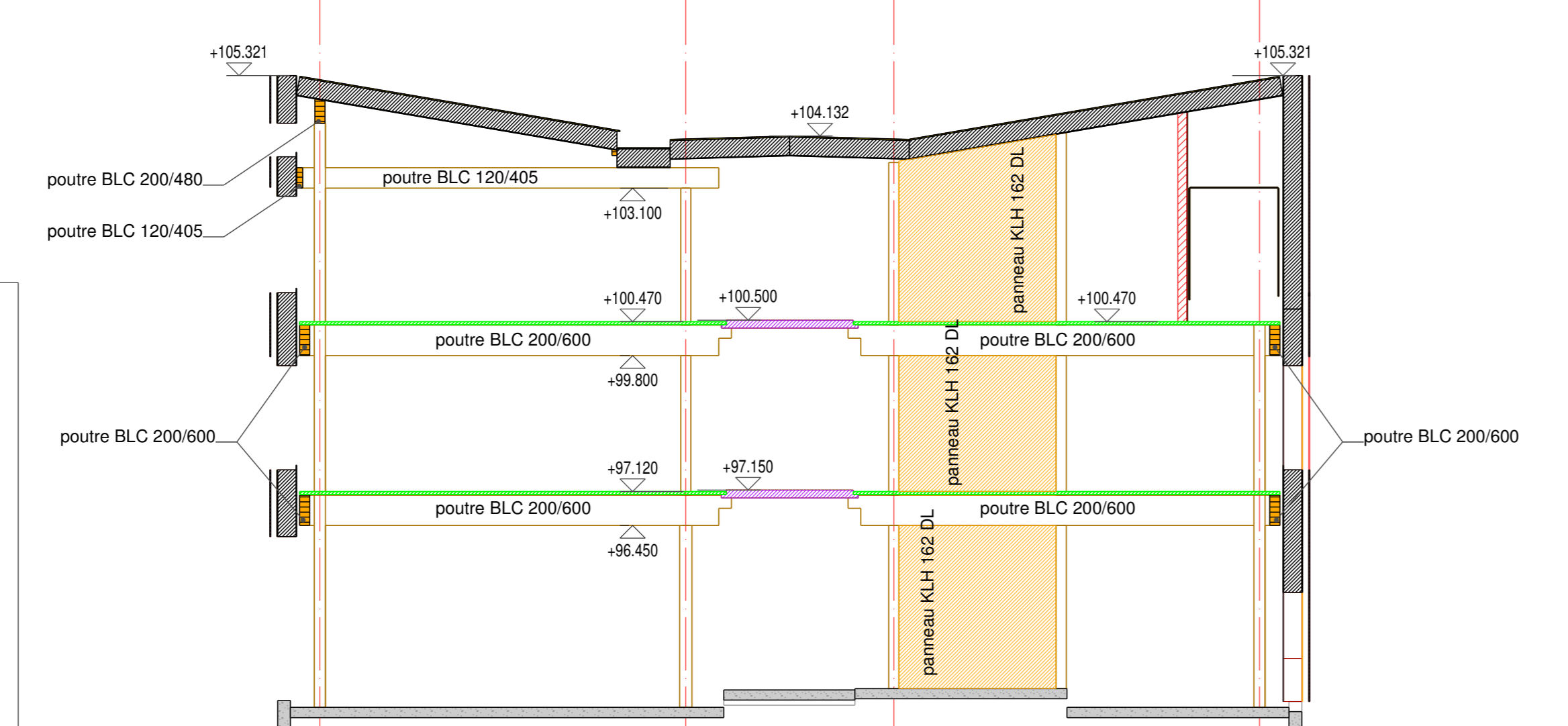
Coupe E
