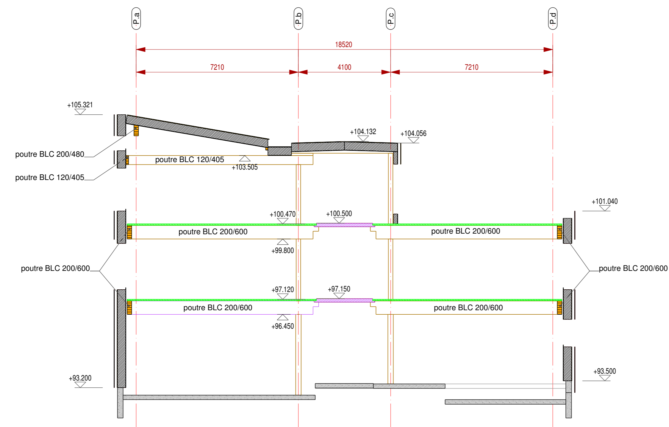
Coupe D
