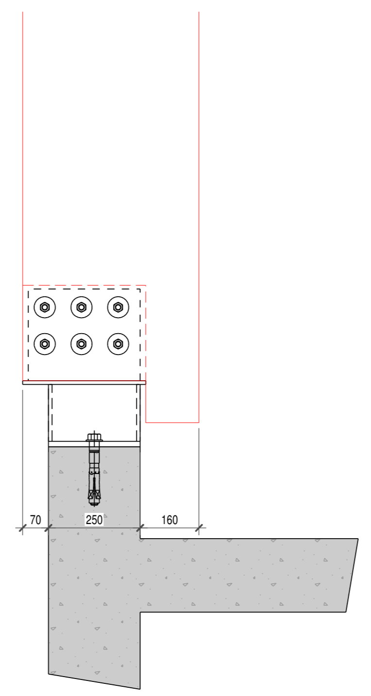
Principe d'appui de poteau sur relevé béton
