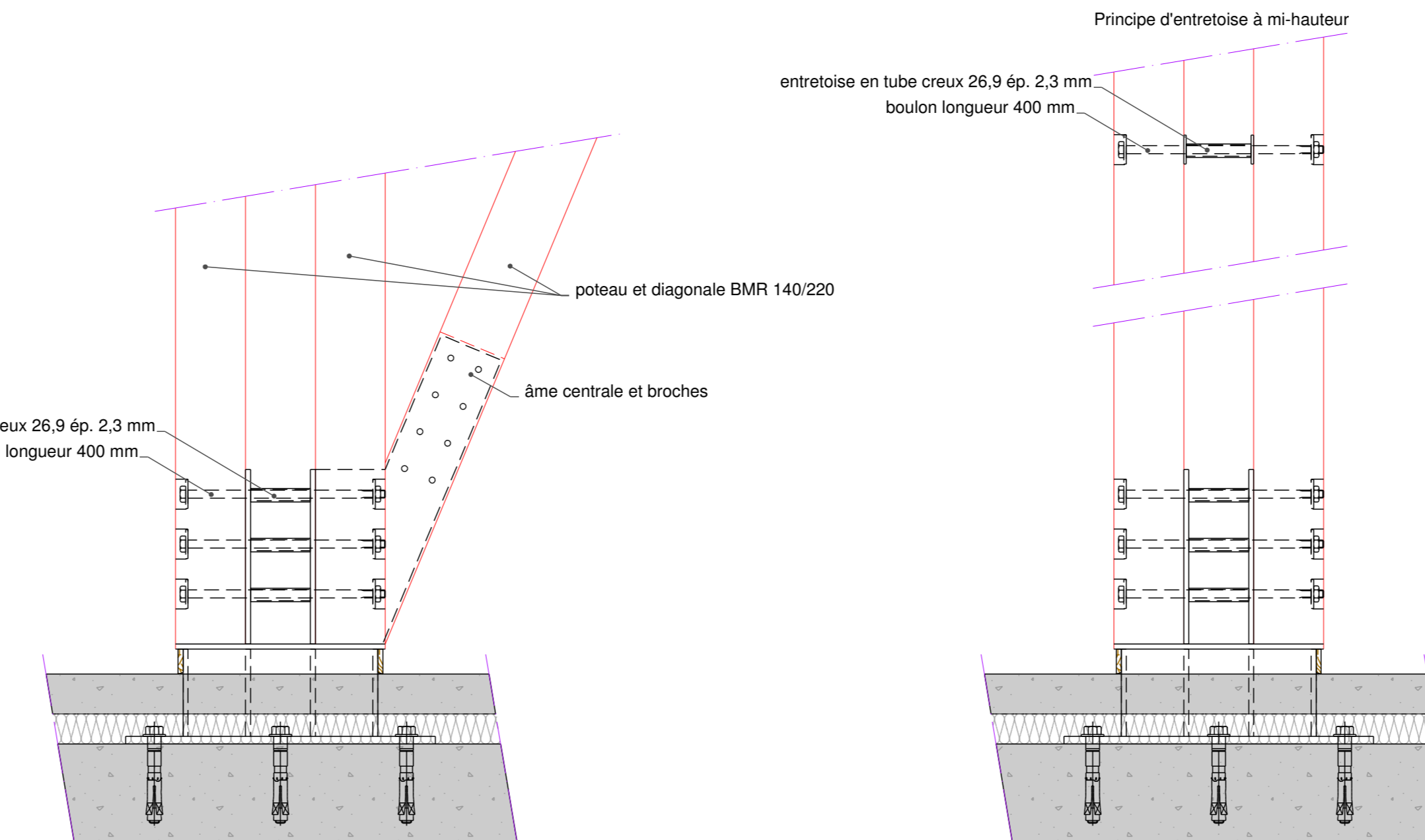
Principe d'assemblage poteaux et diagonales 140/220 (vue de face)
