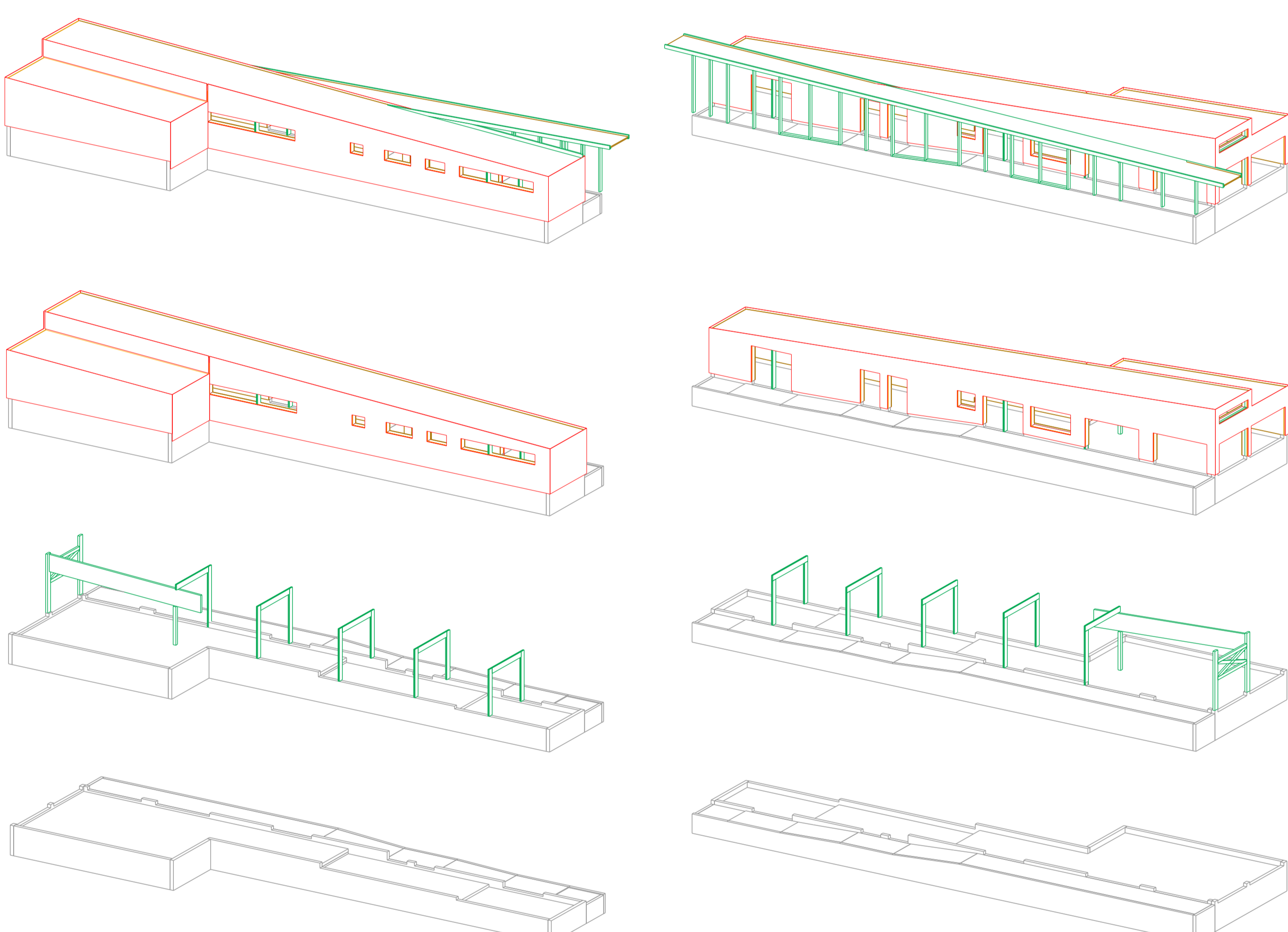
Axonométrie de structure
