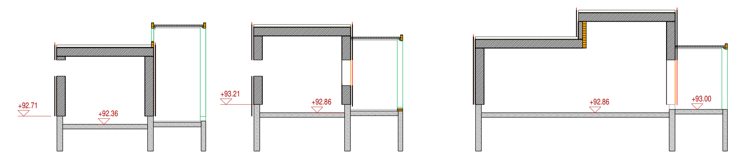
Coupe transversale de structure (1/100e)
