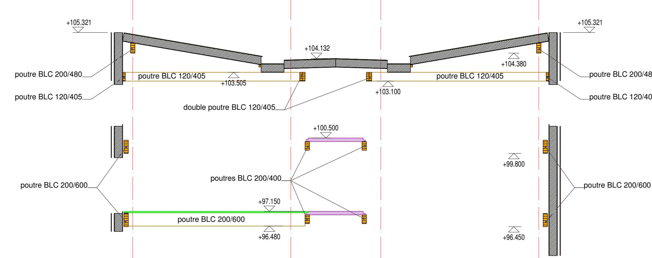
Coupe C
