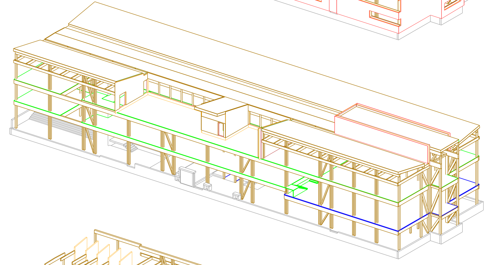
Couverture étanchéité, mur bois R+2
