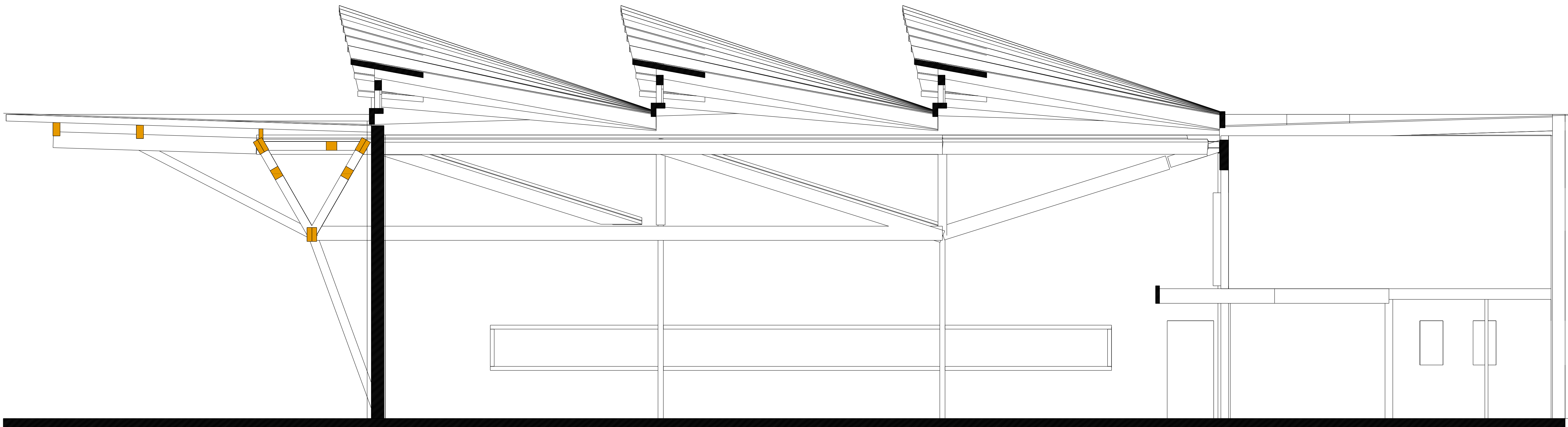
Coupe Nord/Sud 1/50e
