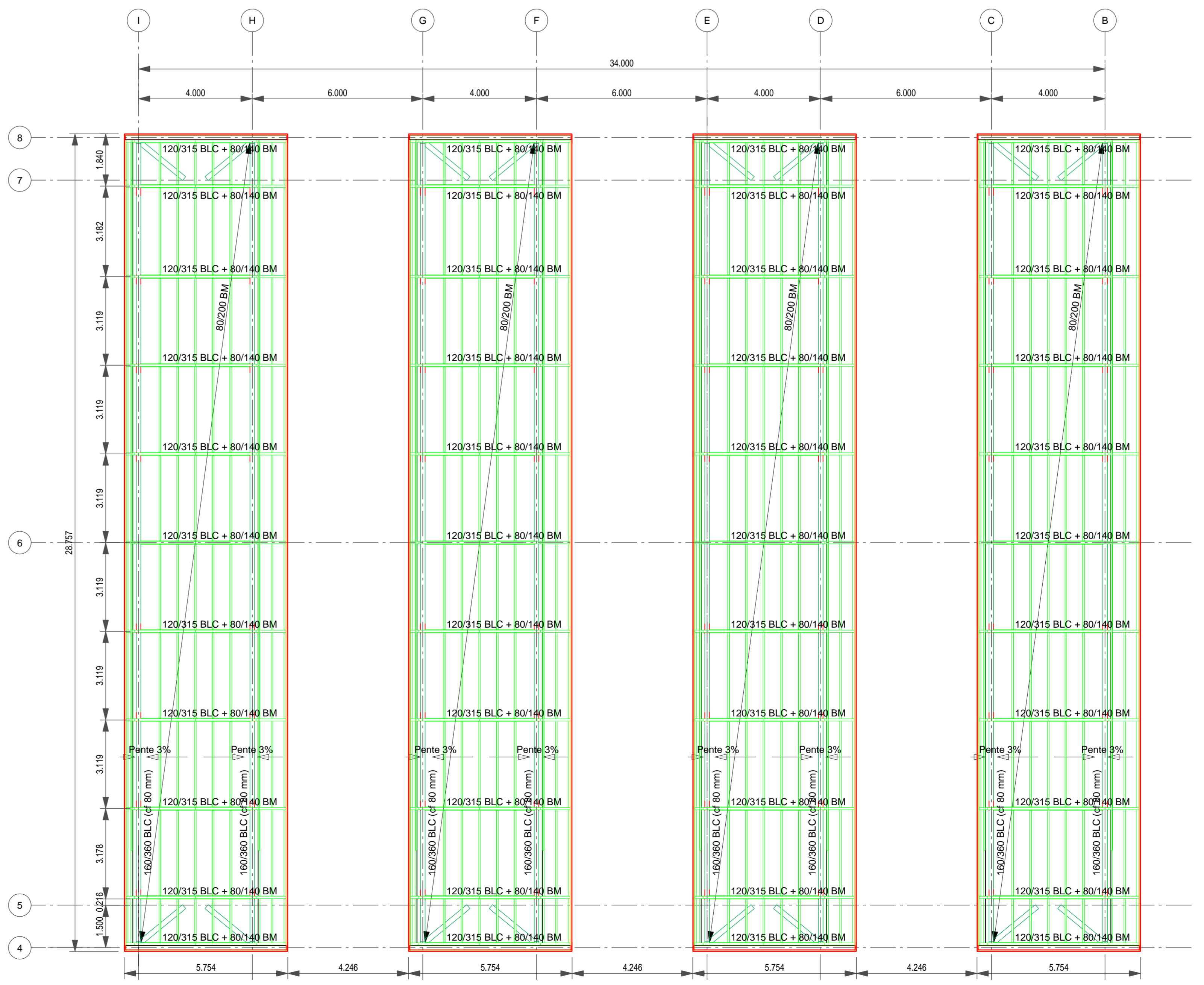
PLAN DE CHARPENTE TOITURES HAUTES SHEDS 1/1000
