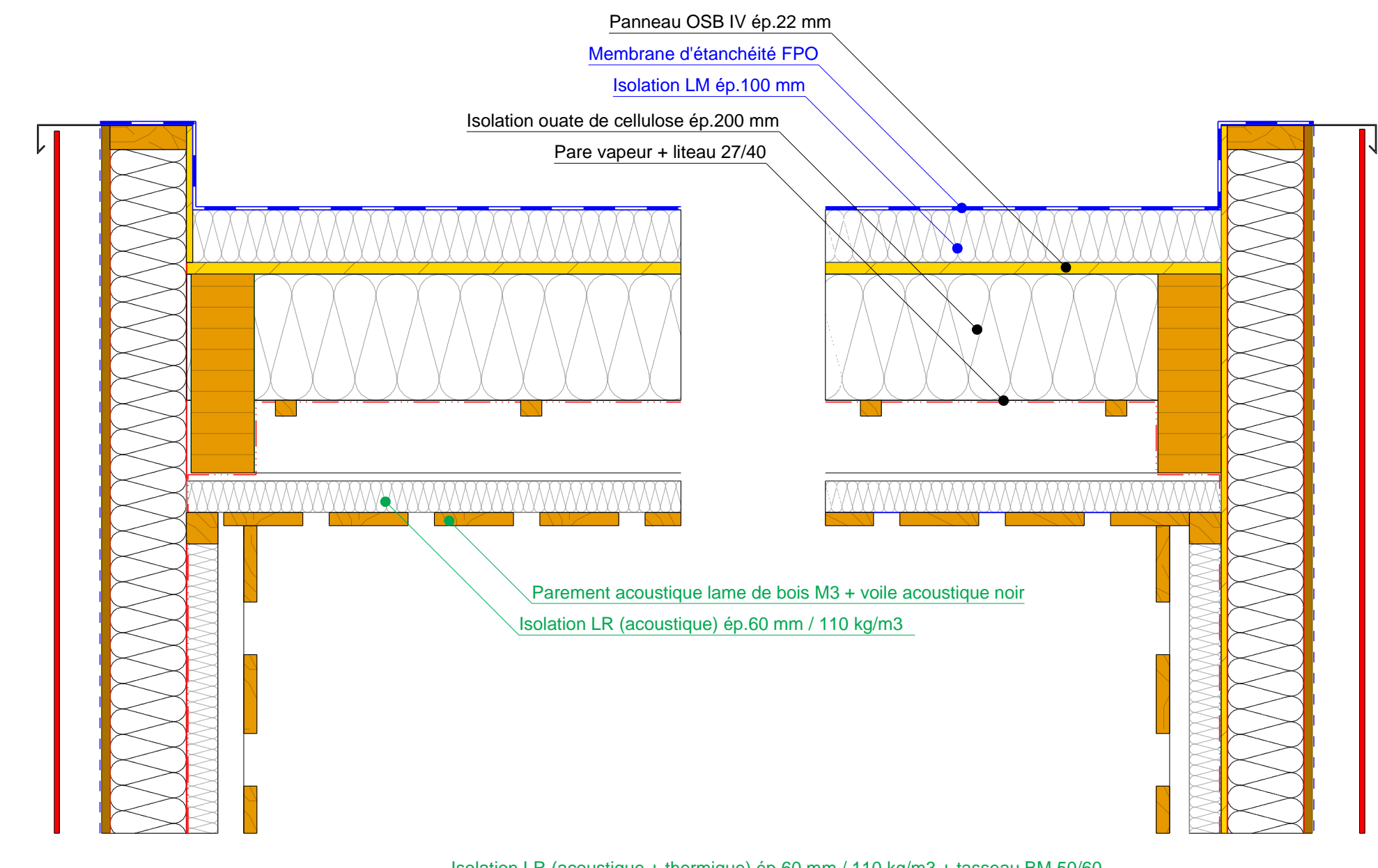
DETAIL COUPE 1-1 1/10e
