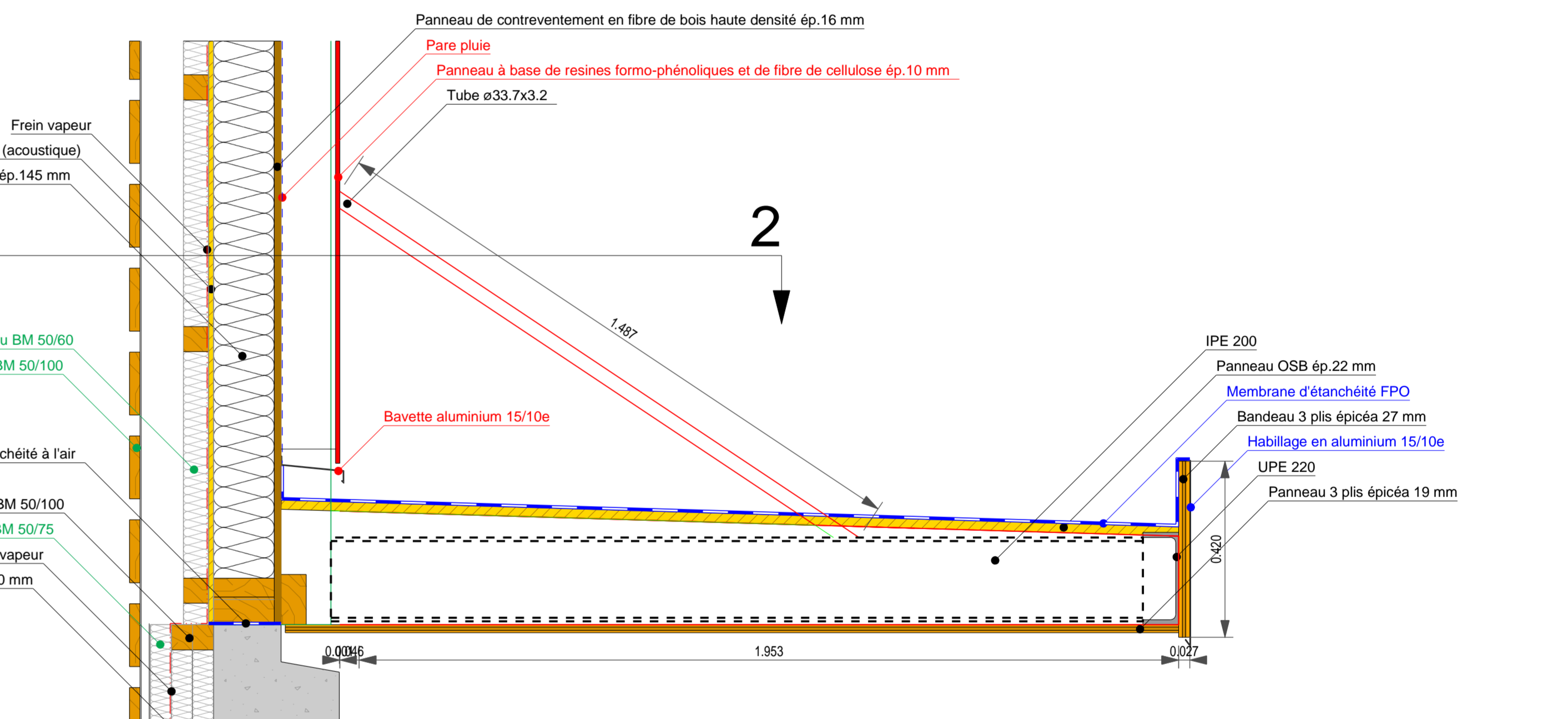
DETAIL COUPE 3-3 1/10e
