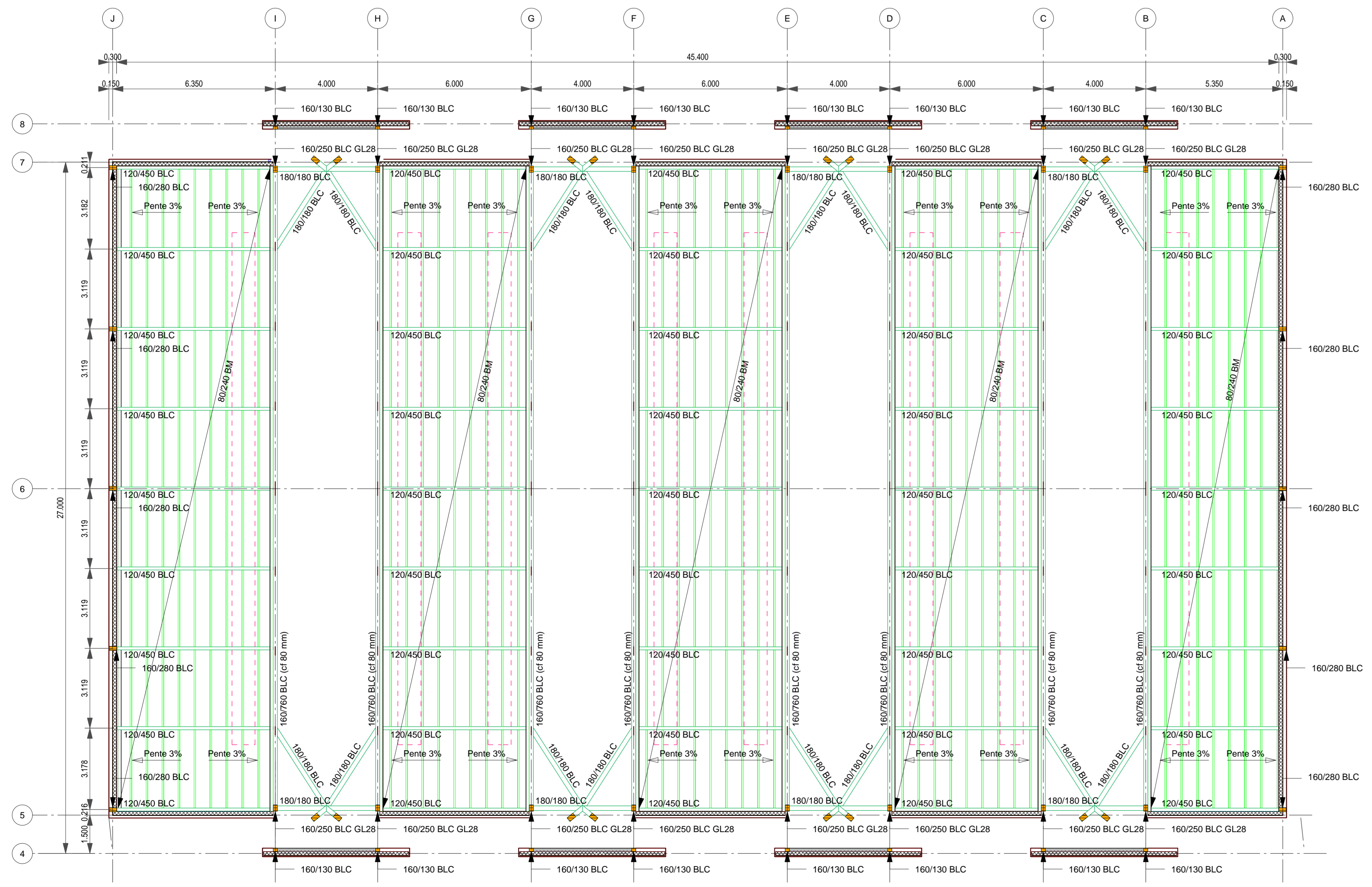
PLAN DE CHARPENTE TOITURES BASSES DES SHEDS 1/1000
