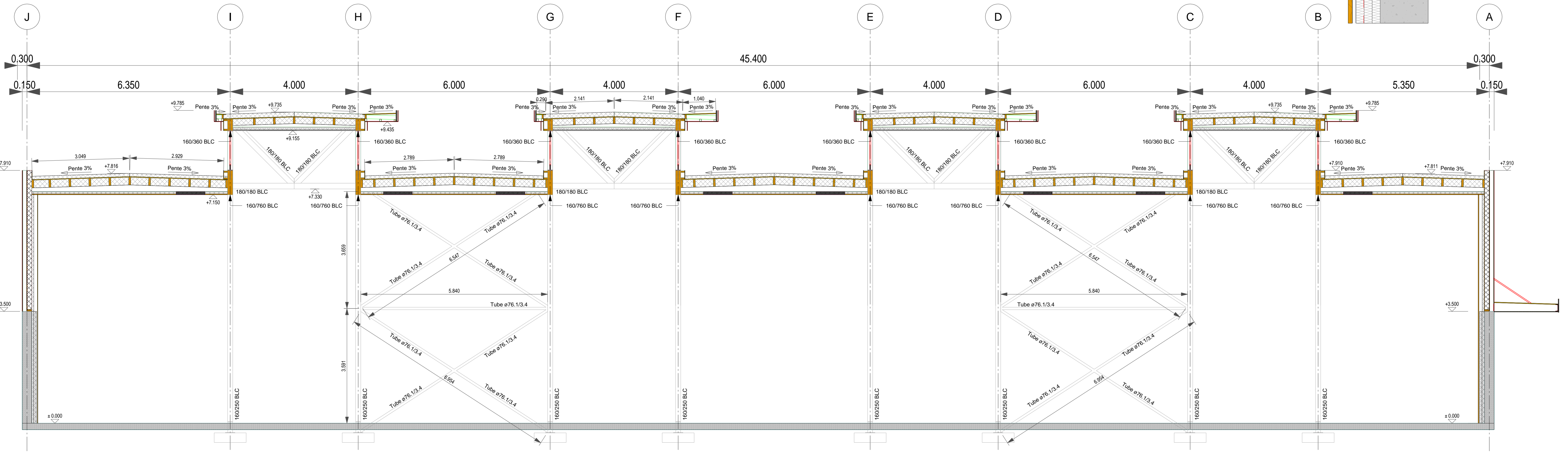
COUPE LONGITUDINALE C-C 1/50e
