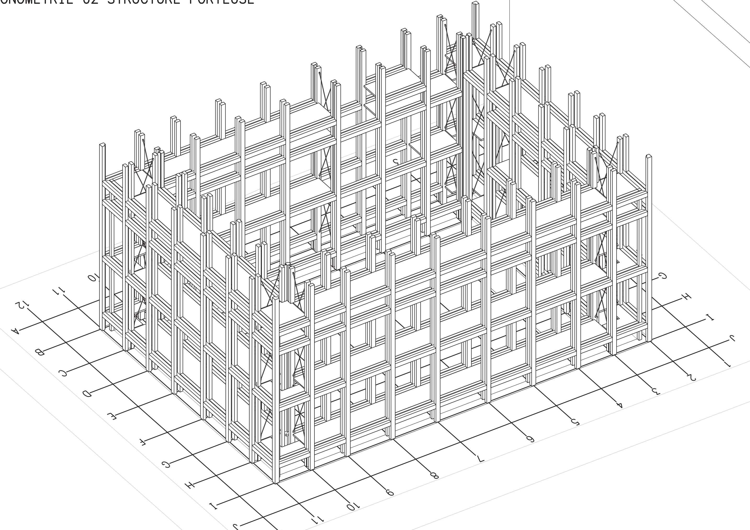
AXONOMETRIE 02 STRUCTURE PORTEUSE
