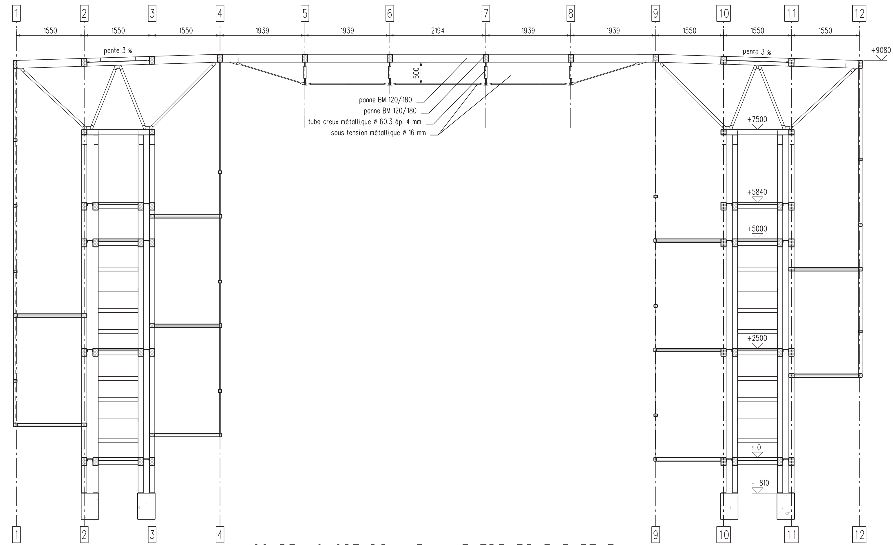
COUPE LONGITUDINALE AA ENTRE FILE E ET F
