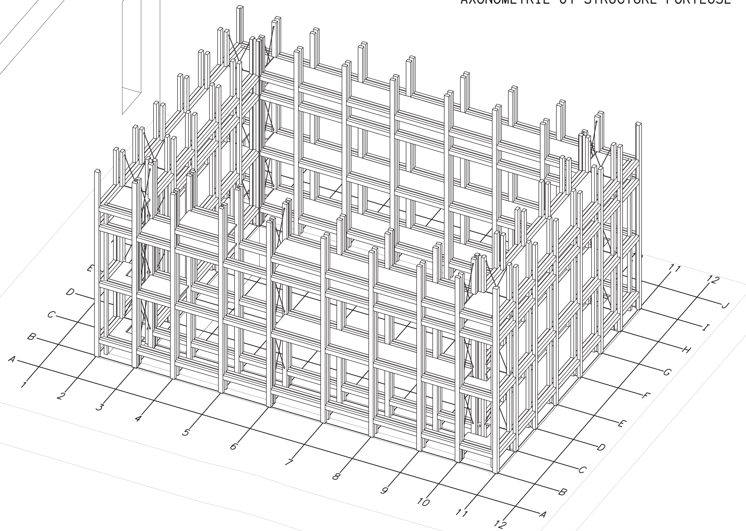
AXONOMETRIE 01 STRUCTURE PORTEUSE
