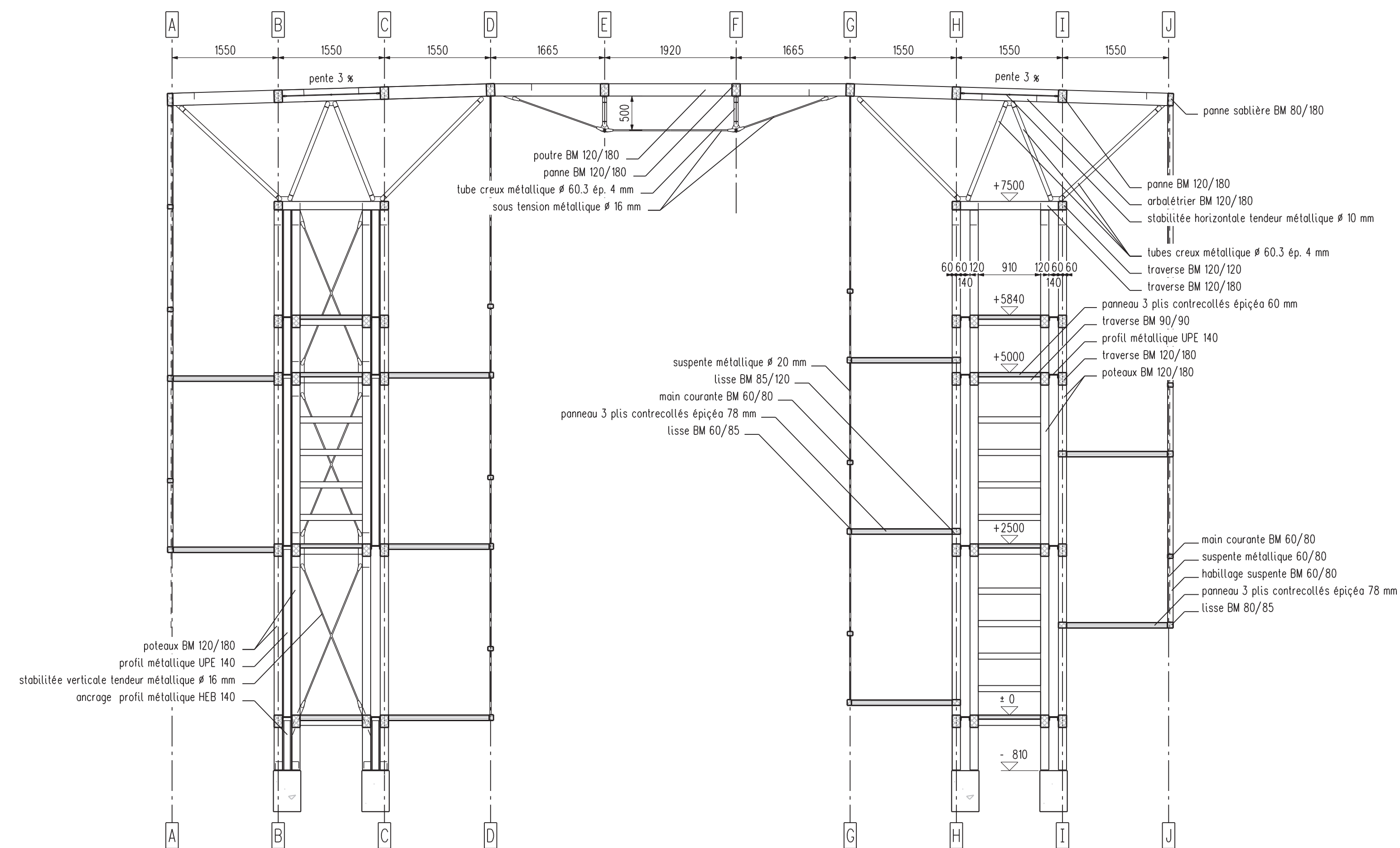
COUPE TRANSVERSALE BB ENTRE FILE 6 ET 7
