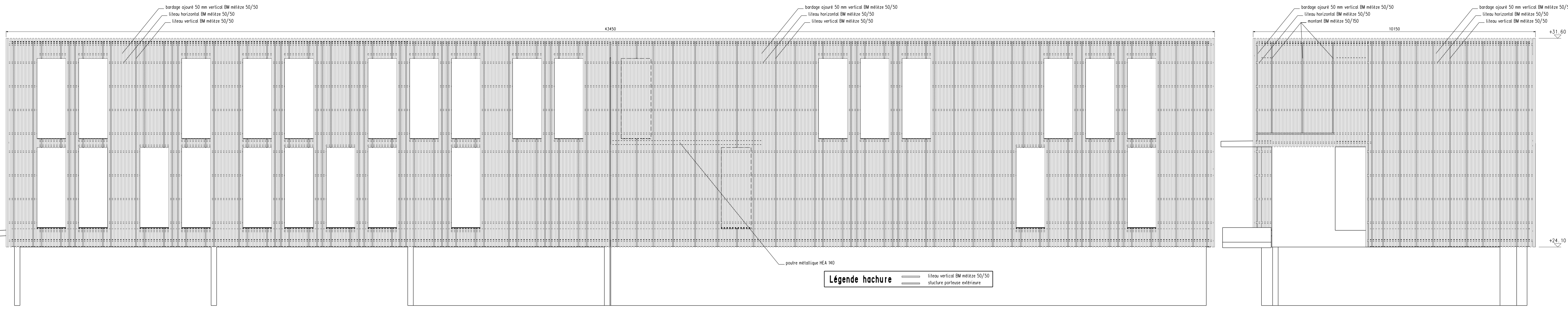
Façade OUEST
