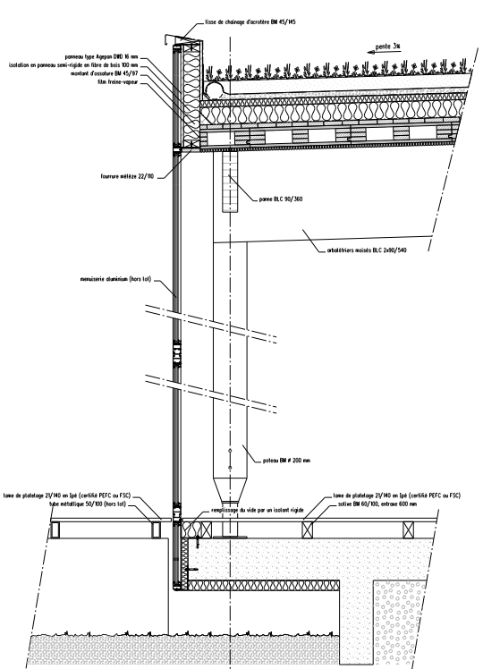
COUPE VERTICALE SUR BAIE VITREE FACADE EST
