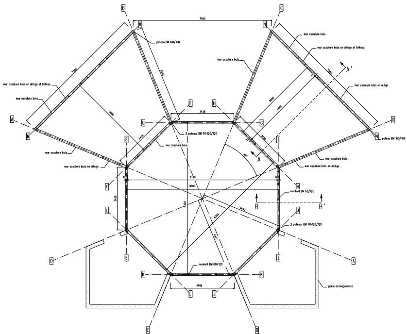
PLAN D'IMPLANTATION DES MURS A OSSATURE BOIS ET DES POTEAUX PORTEURS échelle 1/50e
