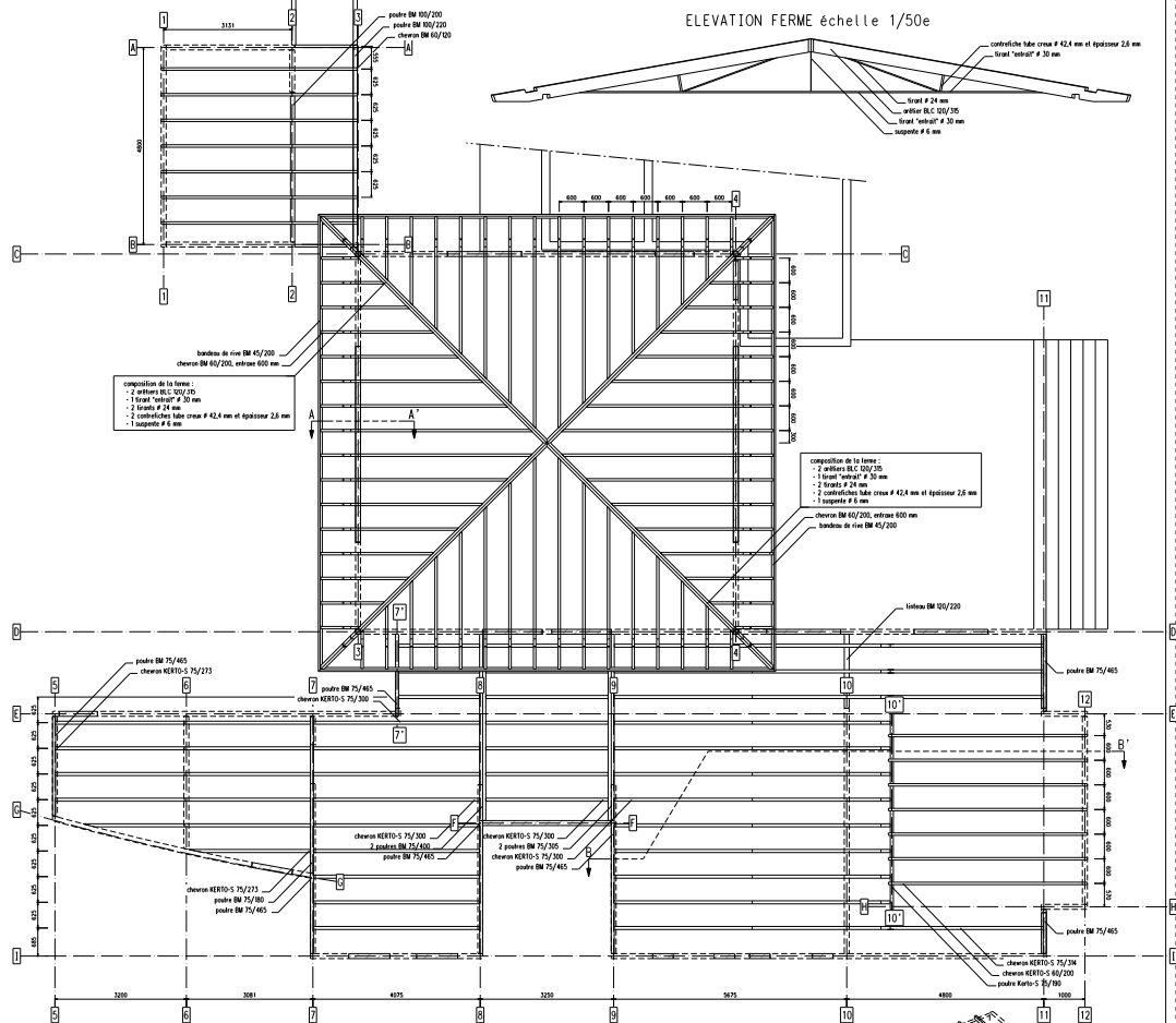
PLAN DE CHARPENTE échelle 1/50e
