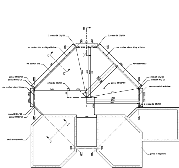
PLAN D'IMPLANTATION DE POTEAUX ET MUR OSSATURE BOIS RDC échelle 1/50e
