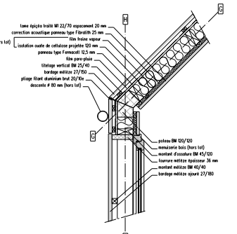
COUPE HORIZONTALE AA' échelle 1/10e
