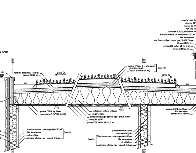
COUPE VERTICALE DE PRINCIPE AA' échelle 1/10e
