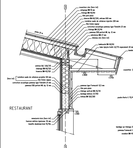
COUPE VERTICALE DE PRINCIPE BB' échelle 1/10e
