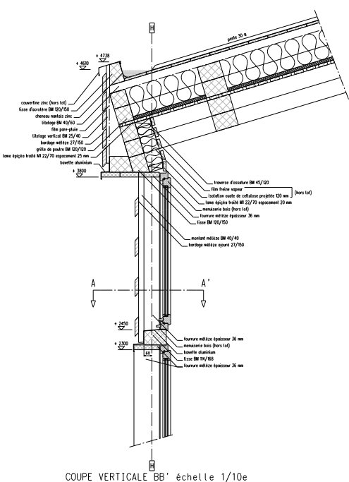
COUPE VERTICALE BB' échelle 1/10e
