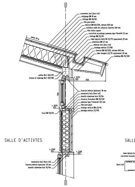
COUPE VERTICALE DE PRINCIPE BB' échelle 1/10e
