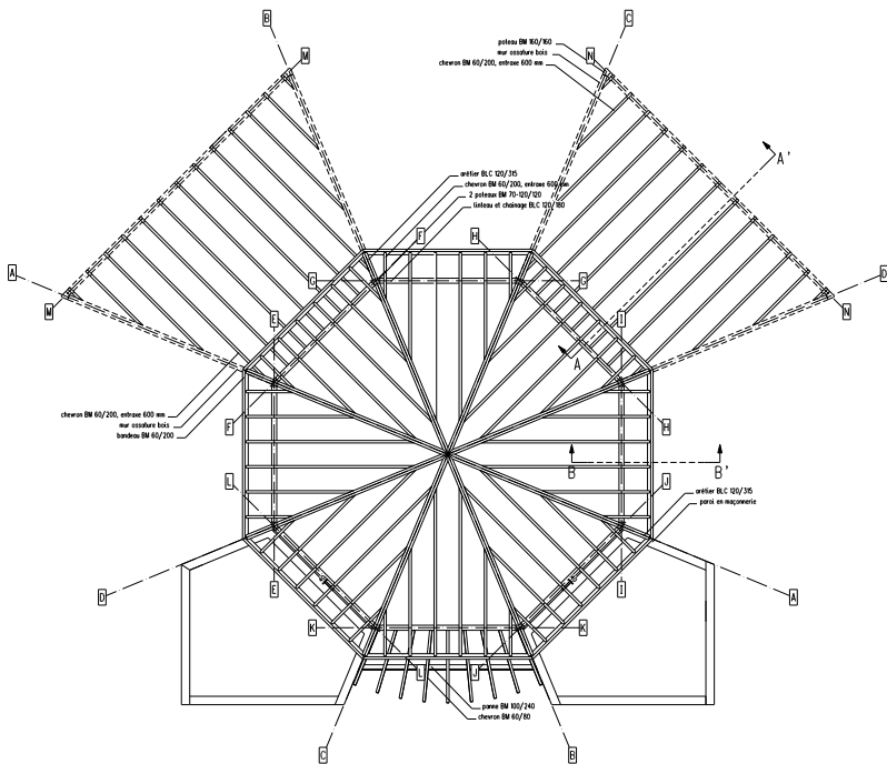
PLAN DE CHARPENTE échelle 1/50e
