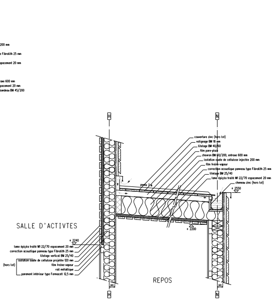
COUPE VERTICALE DE PRINCIPE AA' échelle 1/10e
