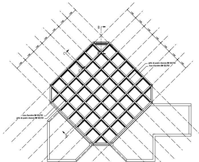
PLAN DE CHARPENTE échelle 1/50e
