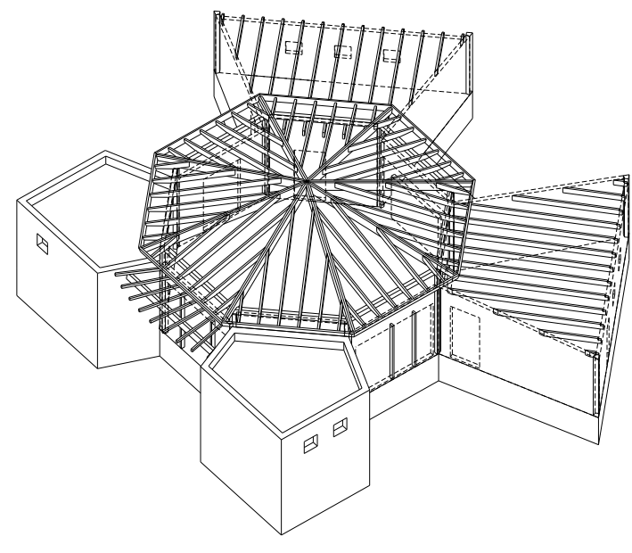
VUE AXONOMETRIQUE DE LA STRUCTURE DE LA CHARPENTE
