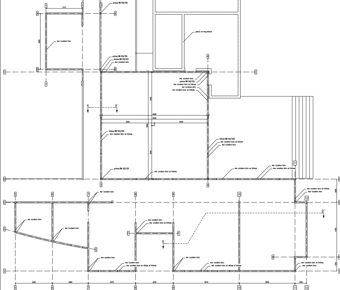
PLAN D'IMPLANTATION DES POTEAUX ET MUR OSSATURE BOIS RDC échelle 1/50e
