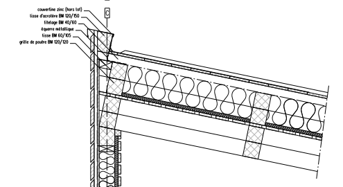
COUPE VERTICALE DD' échelle 1/10e
