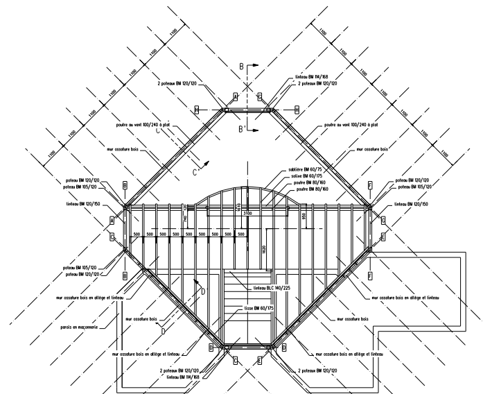
PLAN D'IMPLANTATION DE POTEAUX, MUR OSSATURE BOIS ET STRUCTURE R+1 échelle 1/50e
