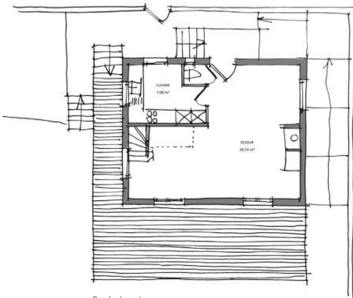
Rez-de-chaussée
