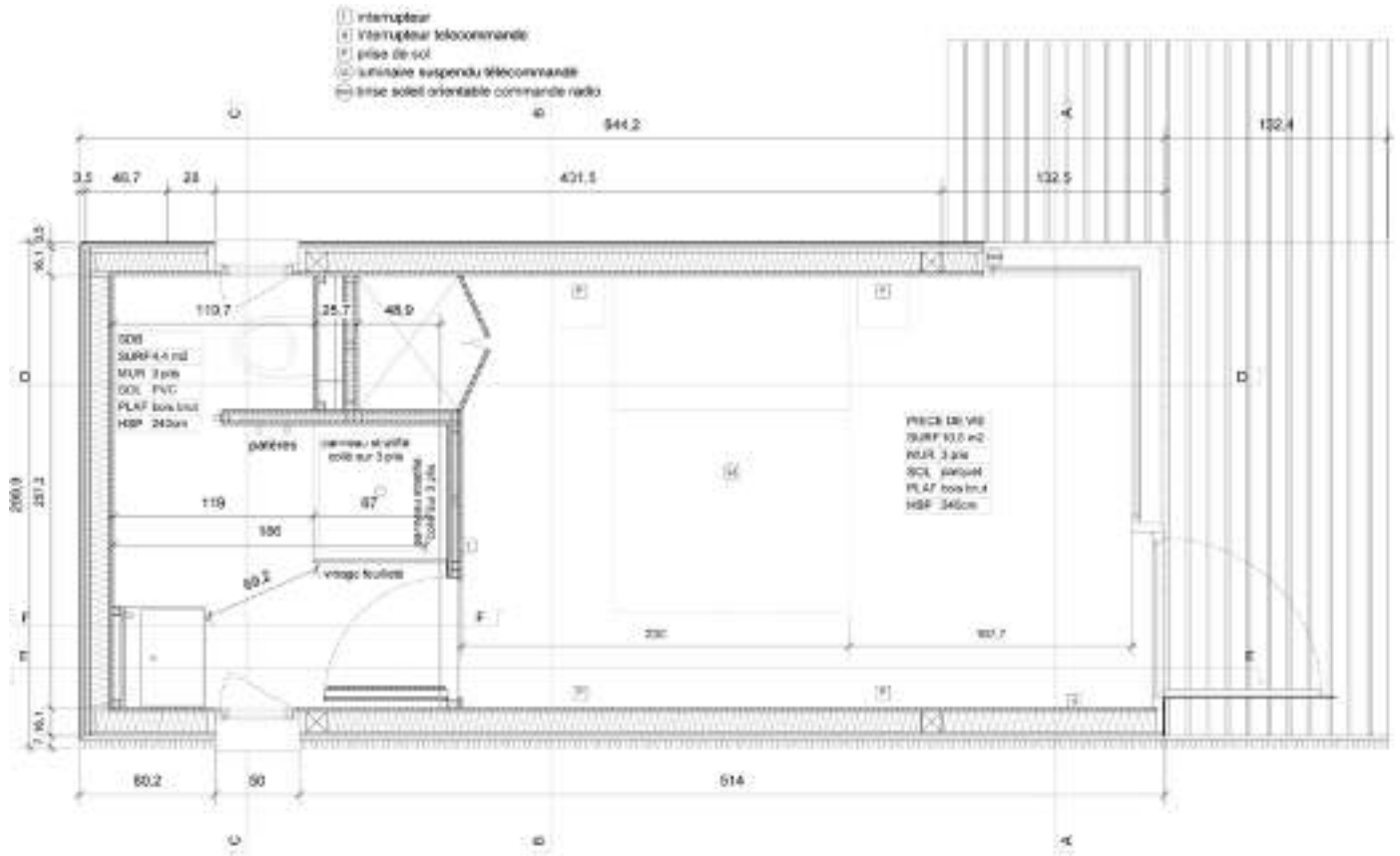
Plan simple
