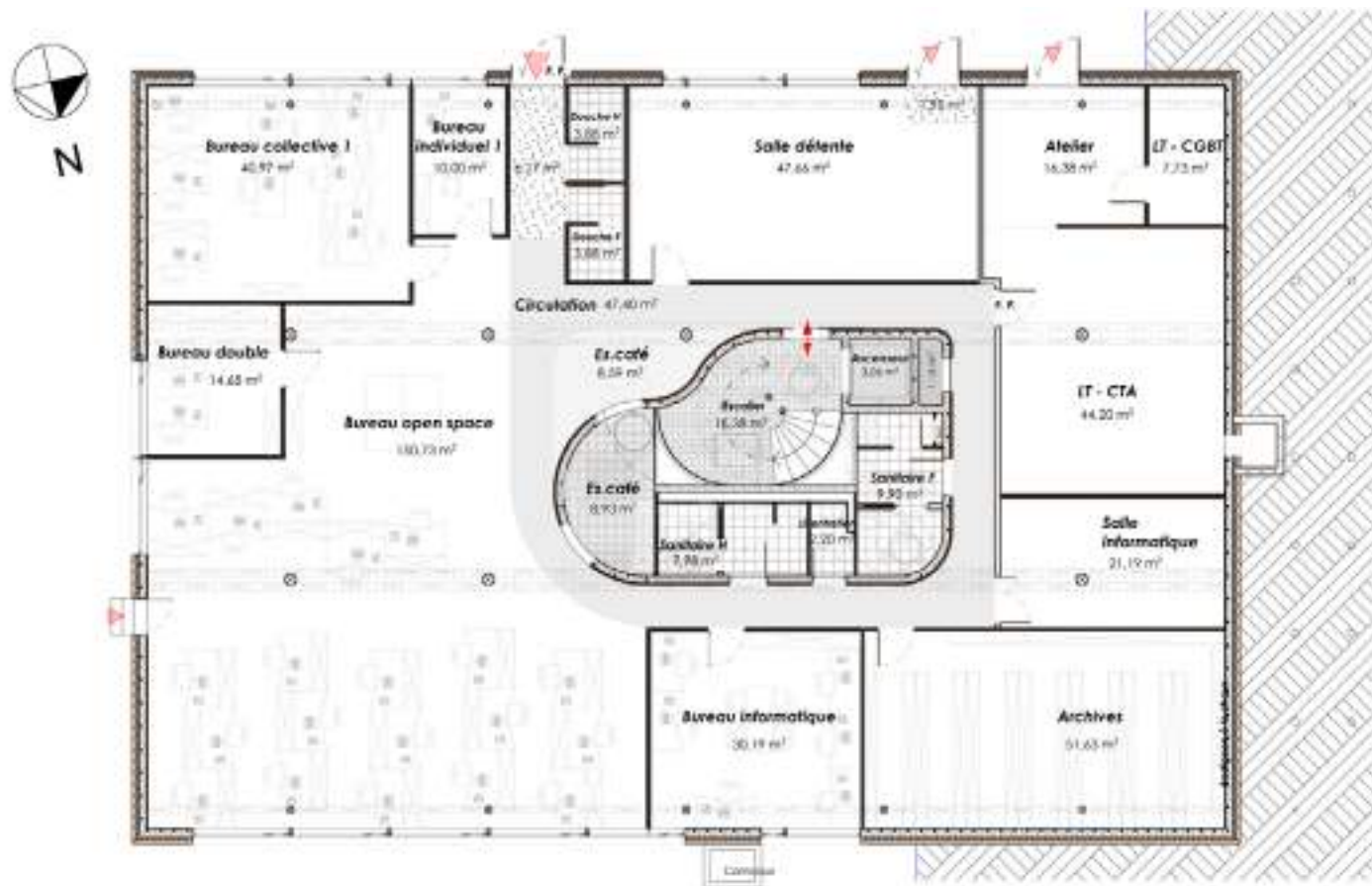
Étage
