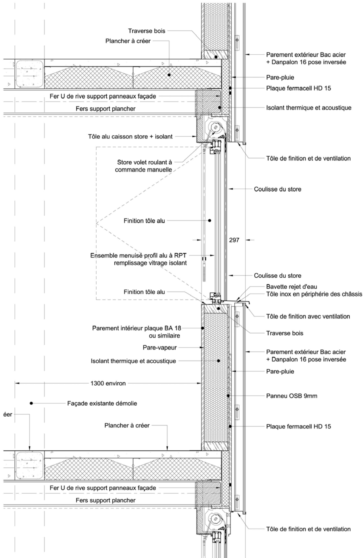
Détail coupe
