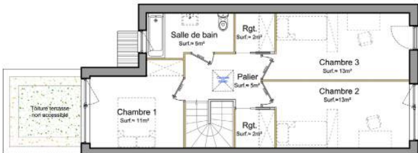
Plan de l'étage
