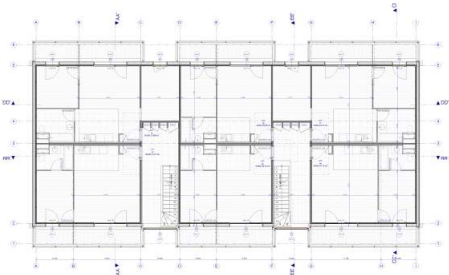
BÂTIMENT B : ÉTAGE 2
