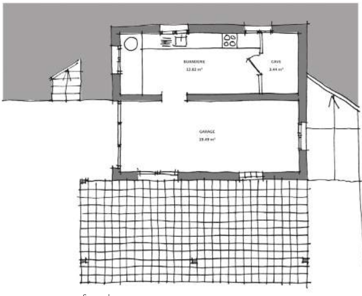
Sous-sol
