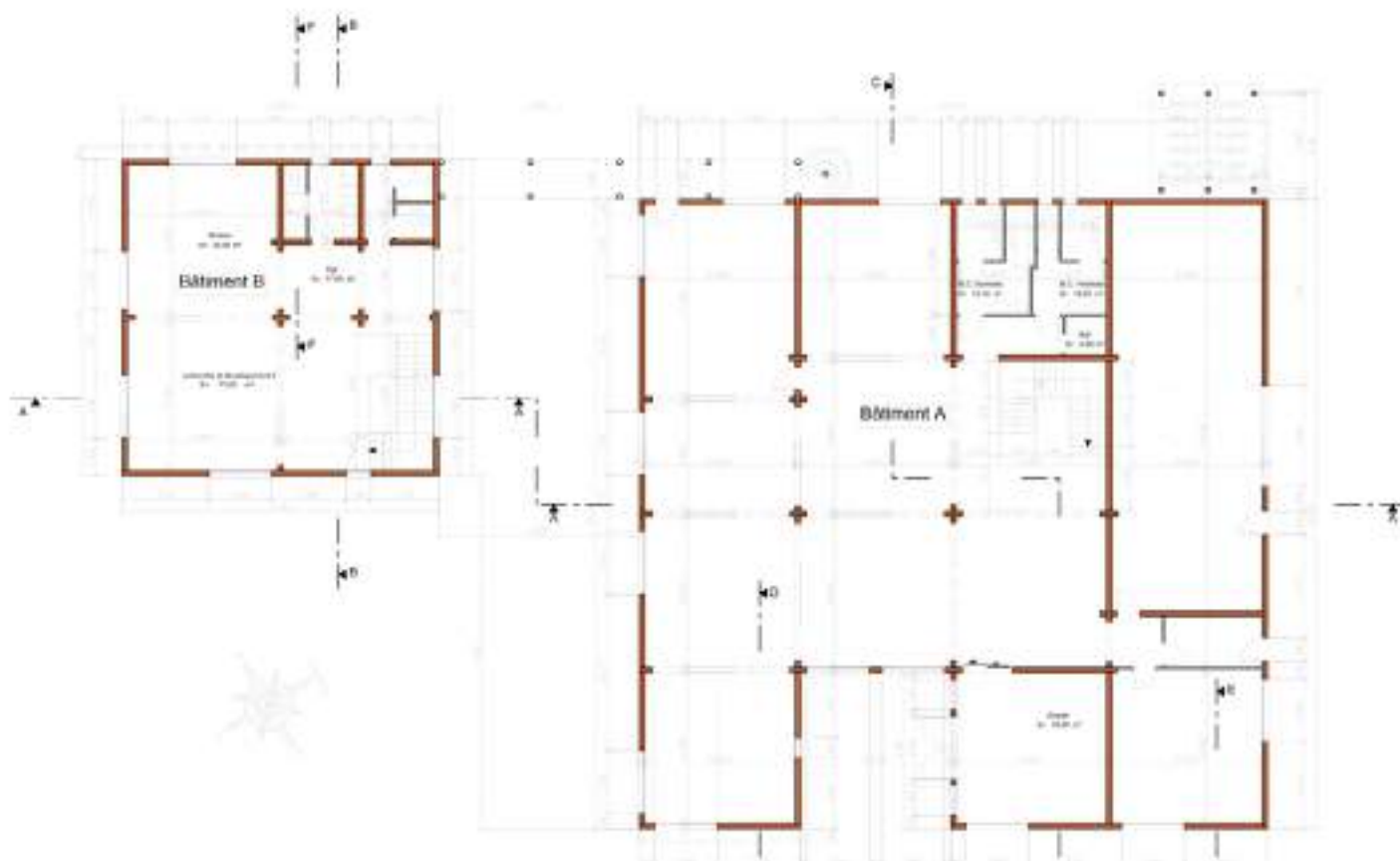
Rez-de-chaussée
