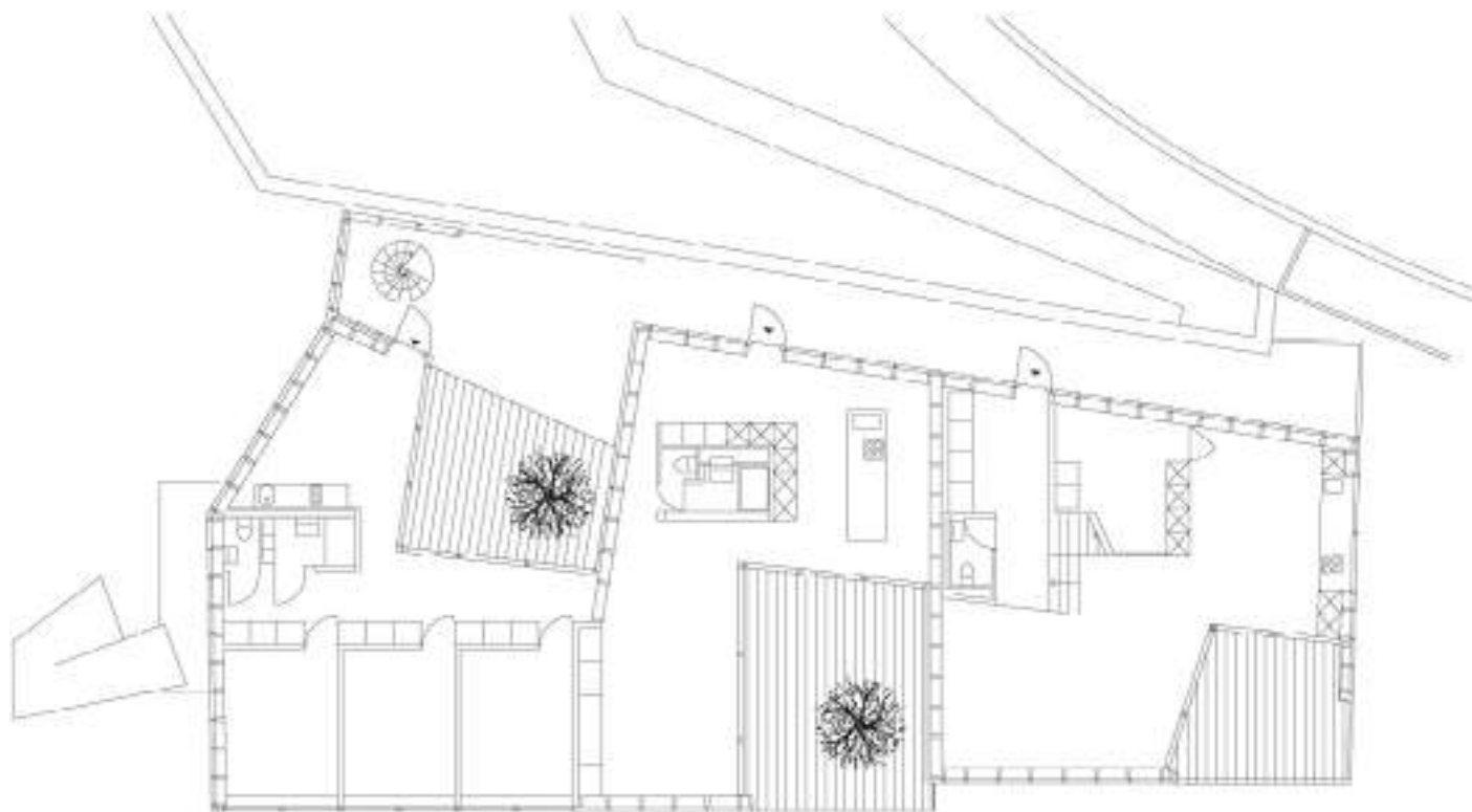
Rehaussement SETIMAC plan niveau entrée éch: 1/200
