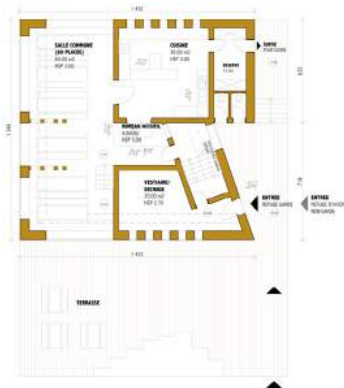
PLAN RDC 1:200 LES COMMUNS/CUISINE 150 m 2
