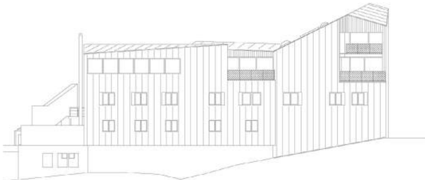
Rehaussement SETIMAC façade Est éch: 1/200
