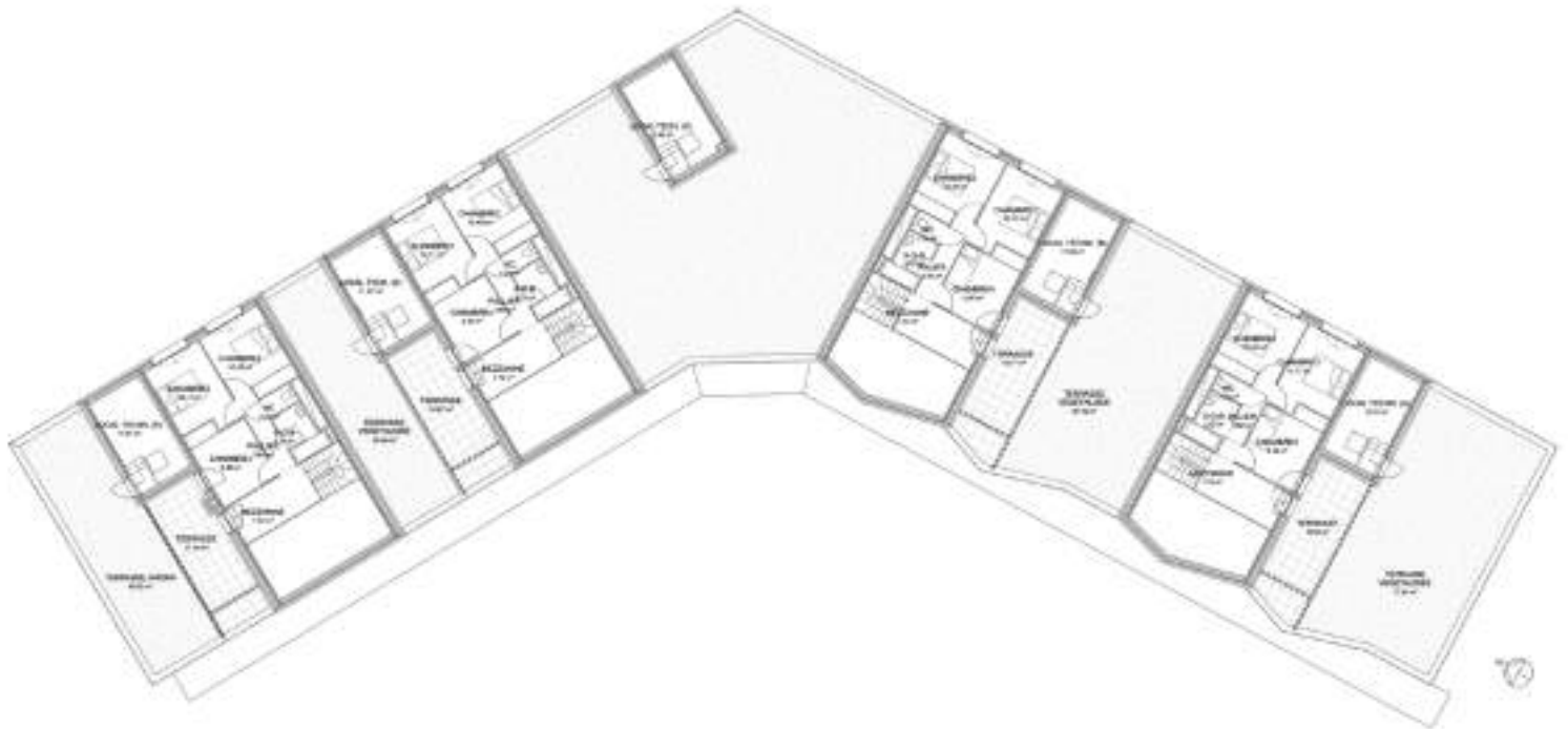
PLAN DU 4 e ÉTAGE DES DUPLEX ET TERRASSES ACCESSIBLES
