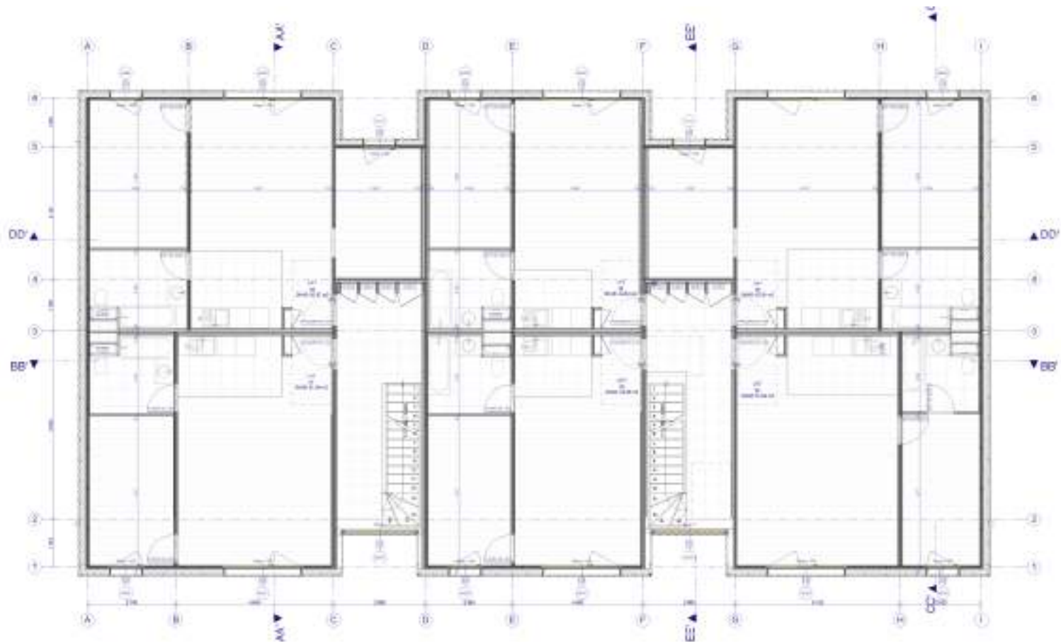
BÂTIMENT B : ÉTAGE 1
