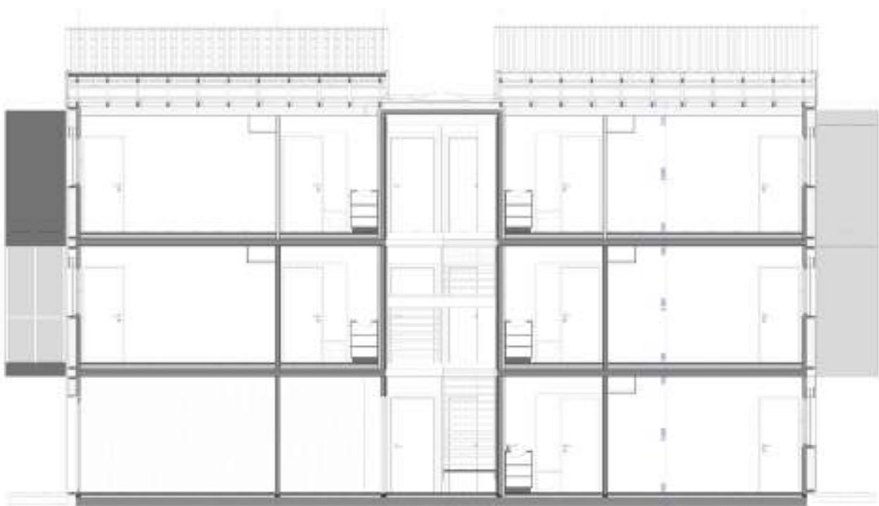
BÂTIMENT A : COUPE
