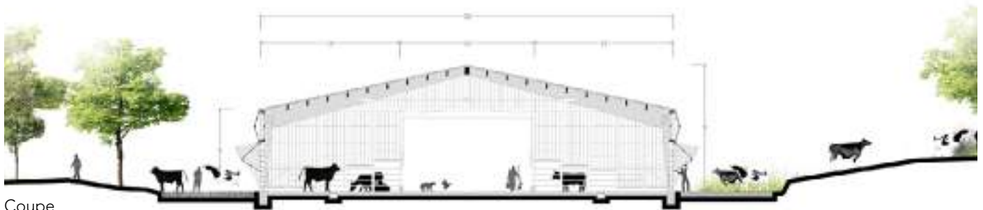
Coupe
