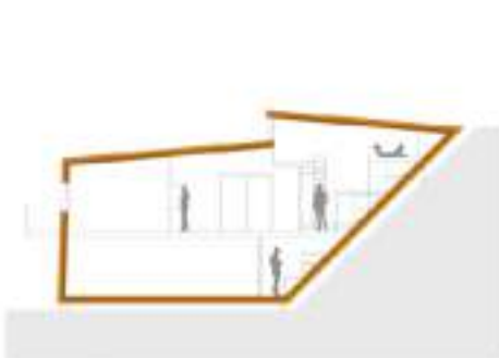
Coupe AA' 1/100
