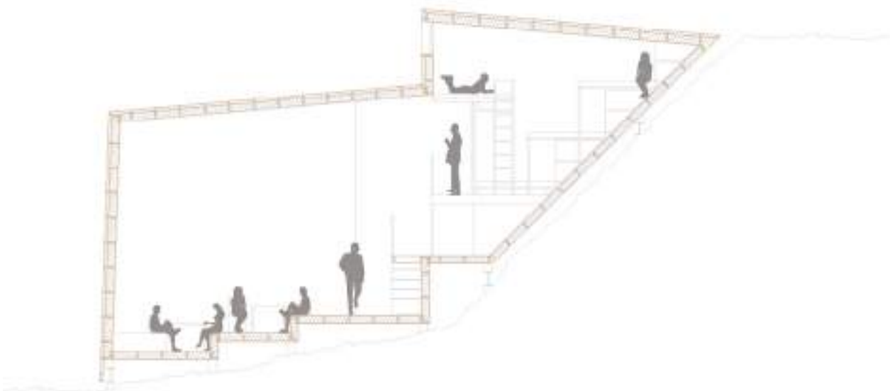
Coupe CC' détail 1/50
