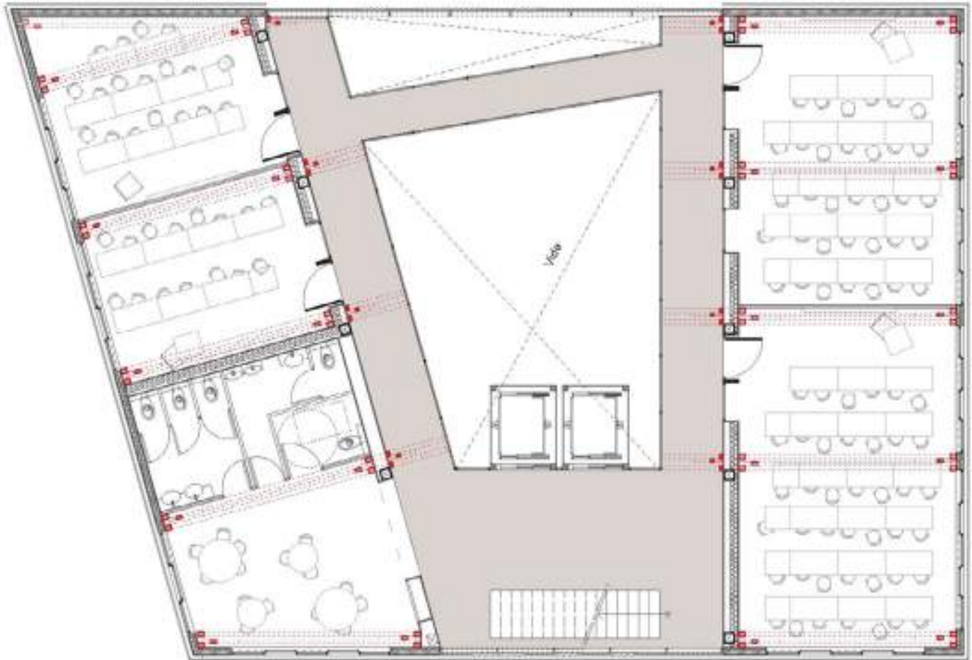
Plan Etage courant
