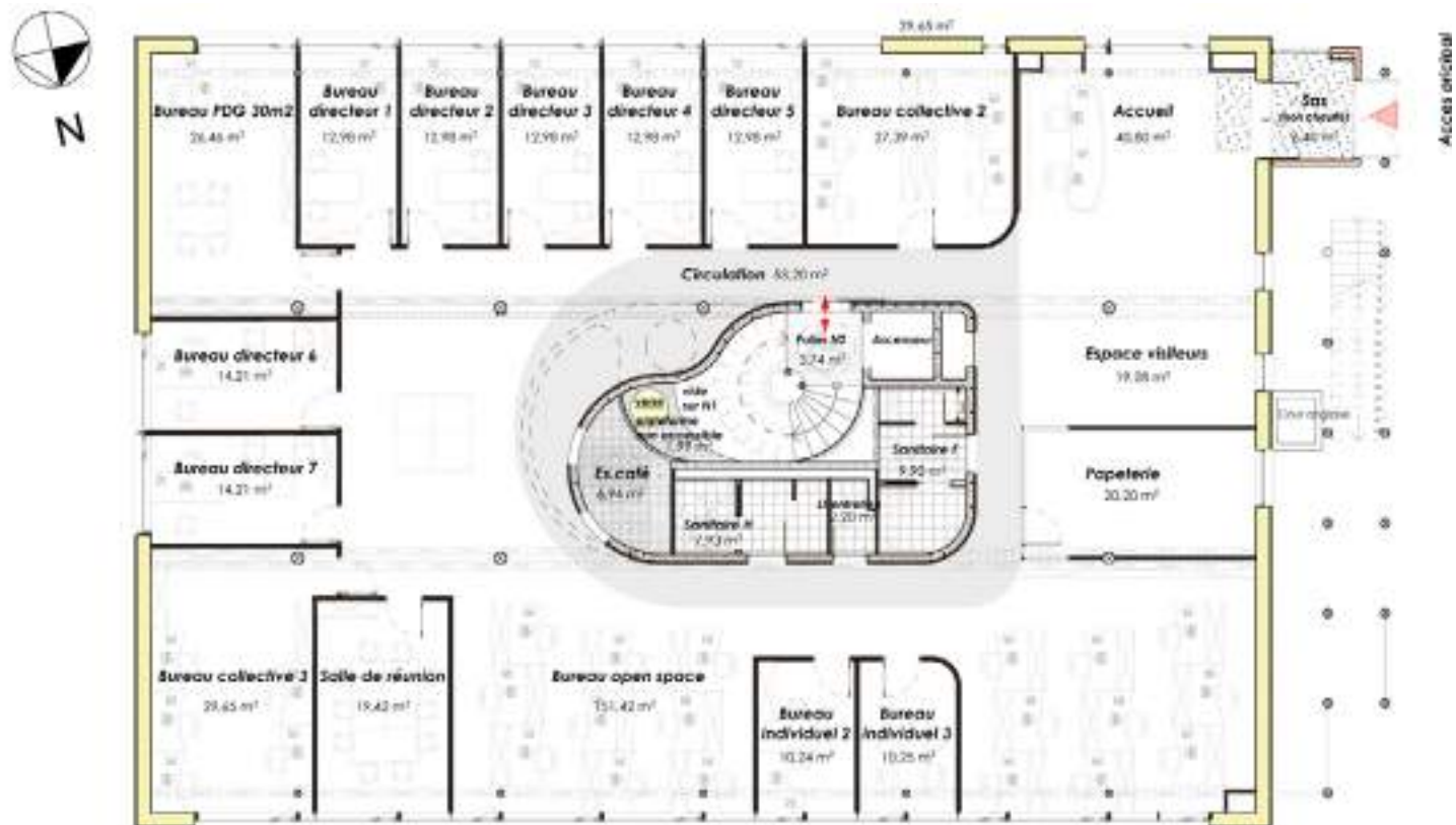
Rez-de-chaussée
