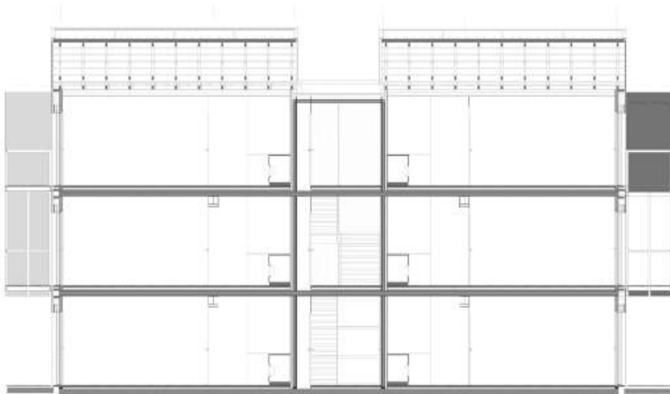
BÂTIMENT A : COUPE
